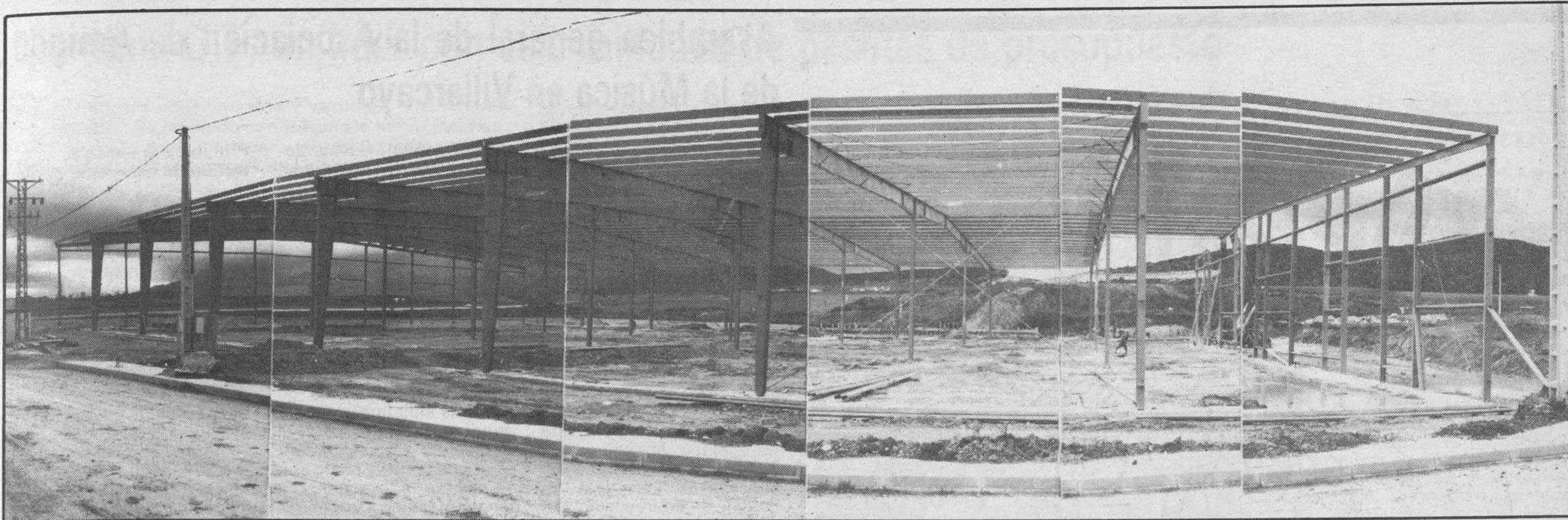
Estructura metálica de la planta fabril.
