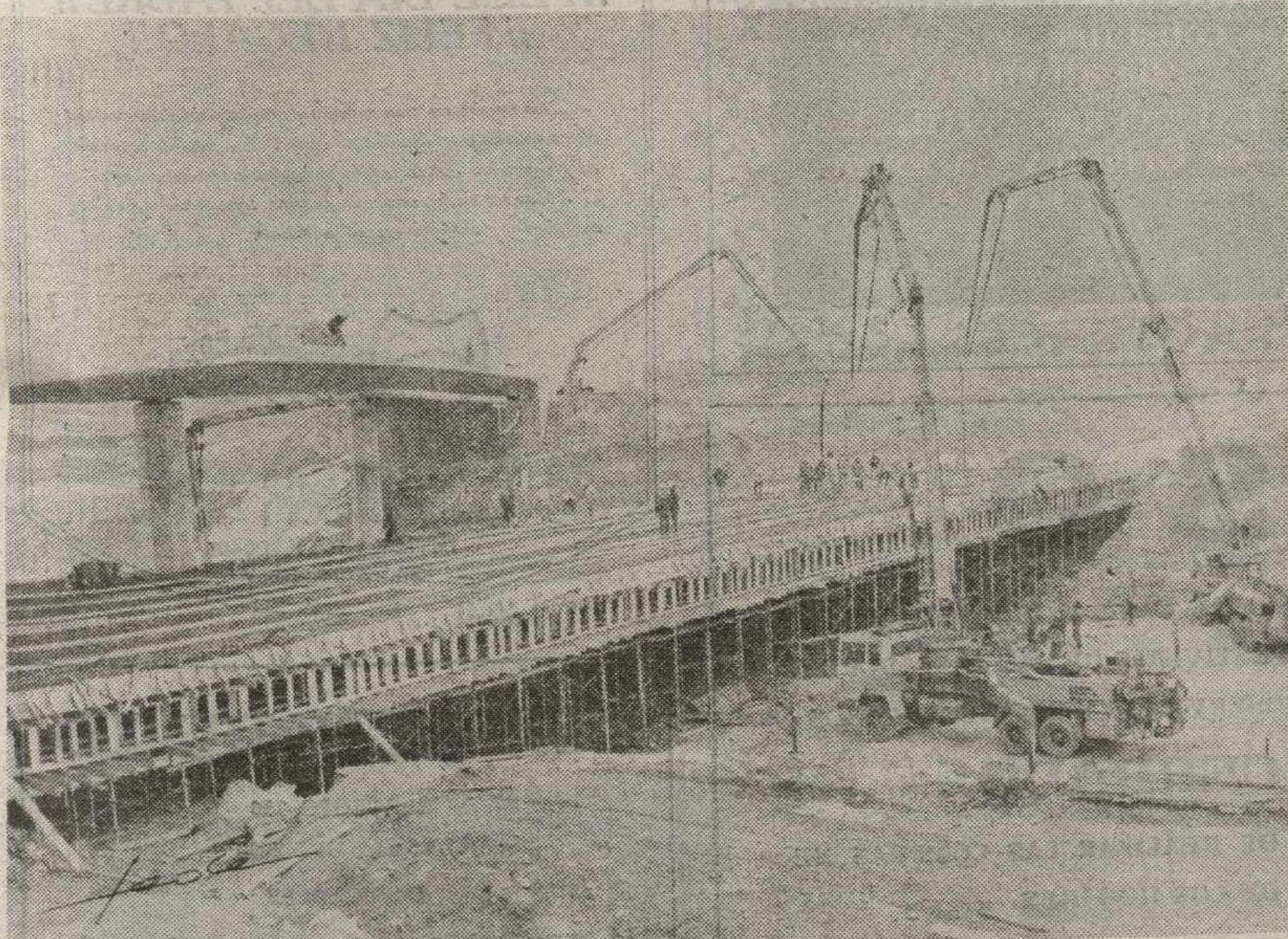
La fotografía nos muestra las obras del nuevo y último puente que completa los enlaces a modo de «scalextric» de la carretera de circunvalación, a la altura del Hostal Landa. Fue hormigonado ayer en una jornada continua de diez horas de duración para rellenar 480 metros cúbicos de hormigón, empleándose cuatro bombas hormigoneras y doce camiones cubas. — (Foto FEDE).
