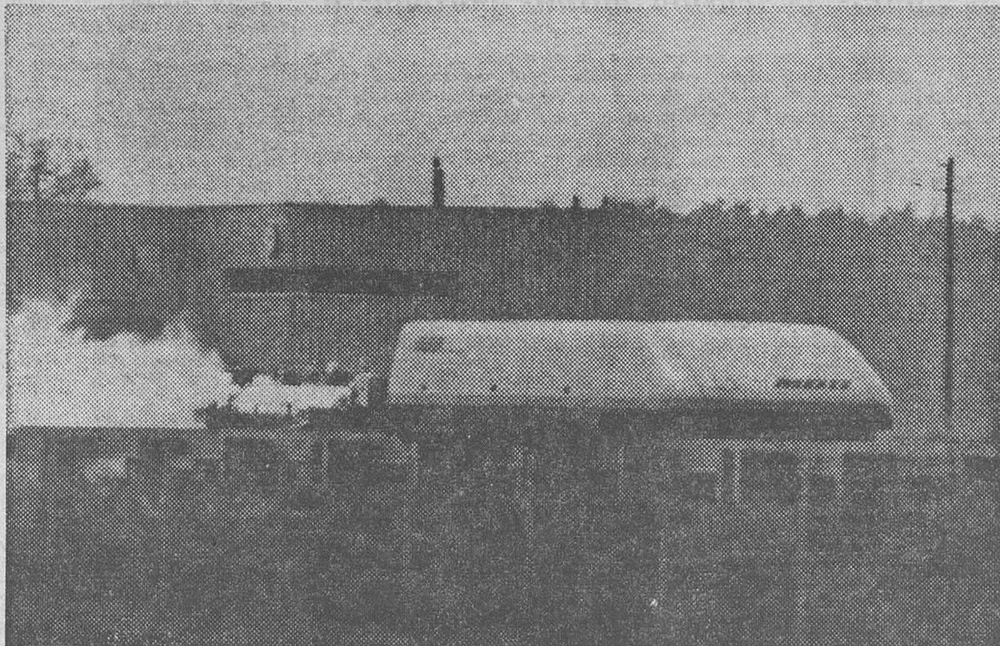
Munich (DaD). — La fotografía capta el instante en que la locomotora de tracción magnética "Komet", fabricada por la industria alemana "MBB" alcanza la velocidad record de 401,3 kilómetros-hora en el circuito experimental de Manching, en las cercanías de Munich (República Federal de Alemania). La locomotora no se desliza sobre el riel, sino que se mueve en estado de suspensión a varios centímetros del riel gracias a un sistema de campos magnéticos. La locomotora es impulsada por un vehículo trineo de vapor. — (Foto DaD/Transrapid EMS).
