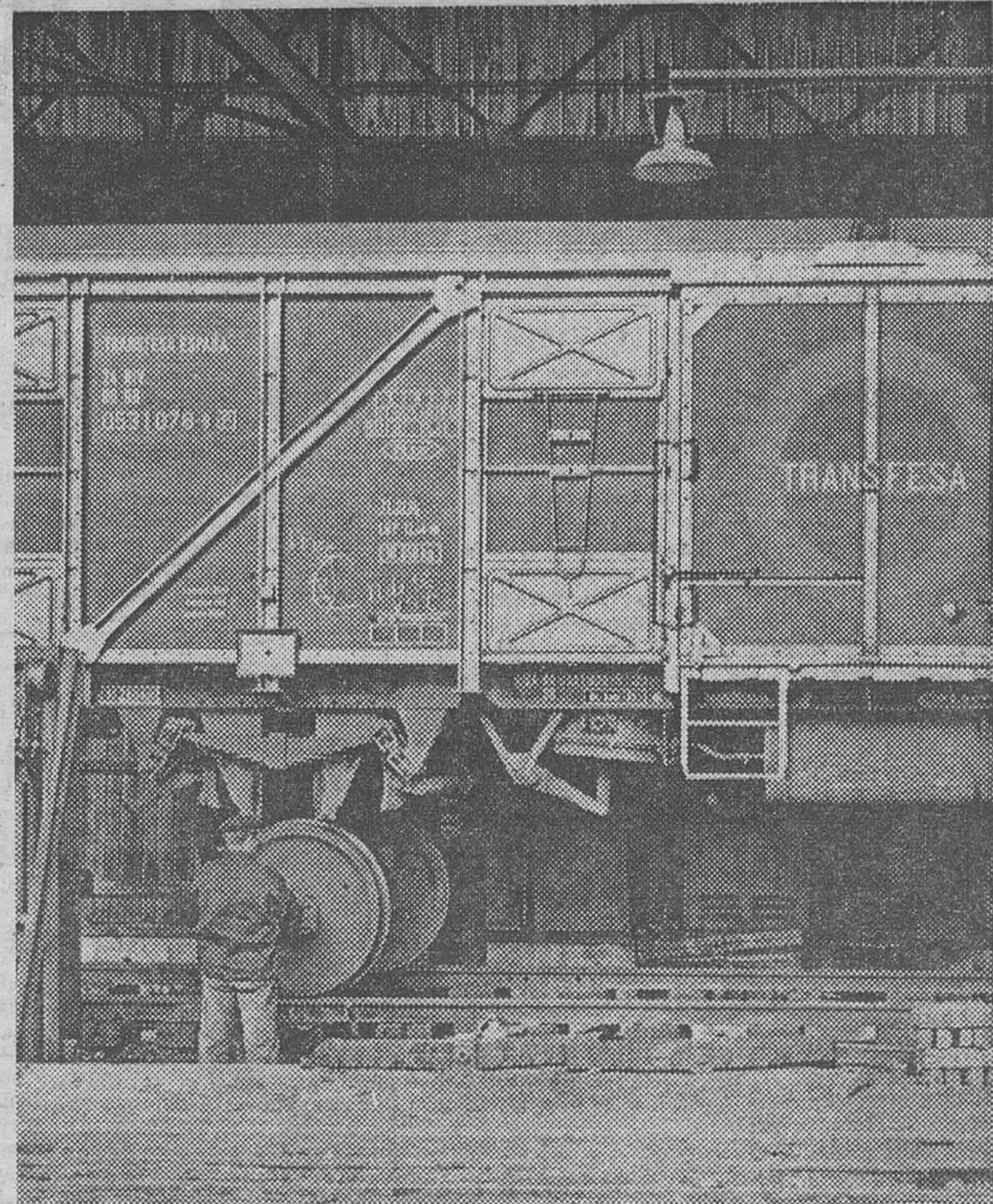
Para hacer más rápido el transporte de contenedores, a través de la frontera hispano-francesa, RENFE, con la colaboración de Transesa ha construido estaciones para el paso del ancho de vía español al europeo. Se han construido vagones con ejes intercambiables. De esta manera, la operación se efectúa en pocos minutos, salvando una diferencia que hasta ahora venía retrasando la entrega del material transportado.
