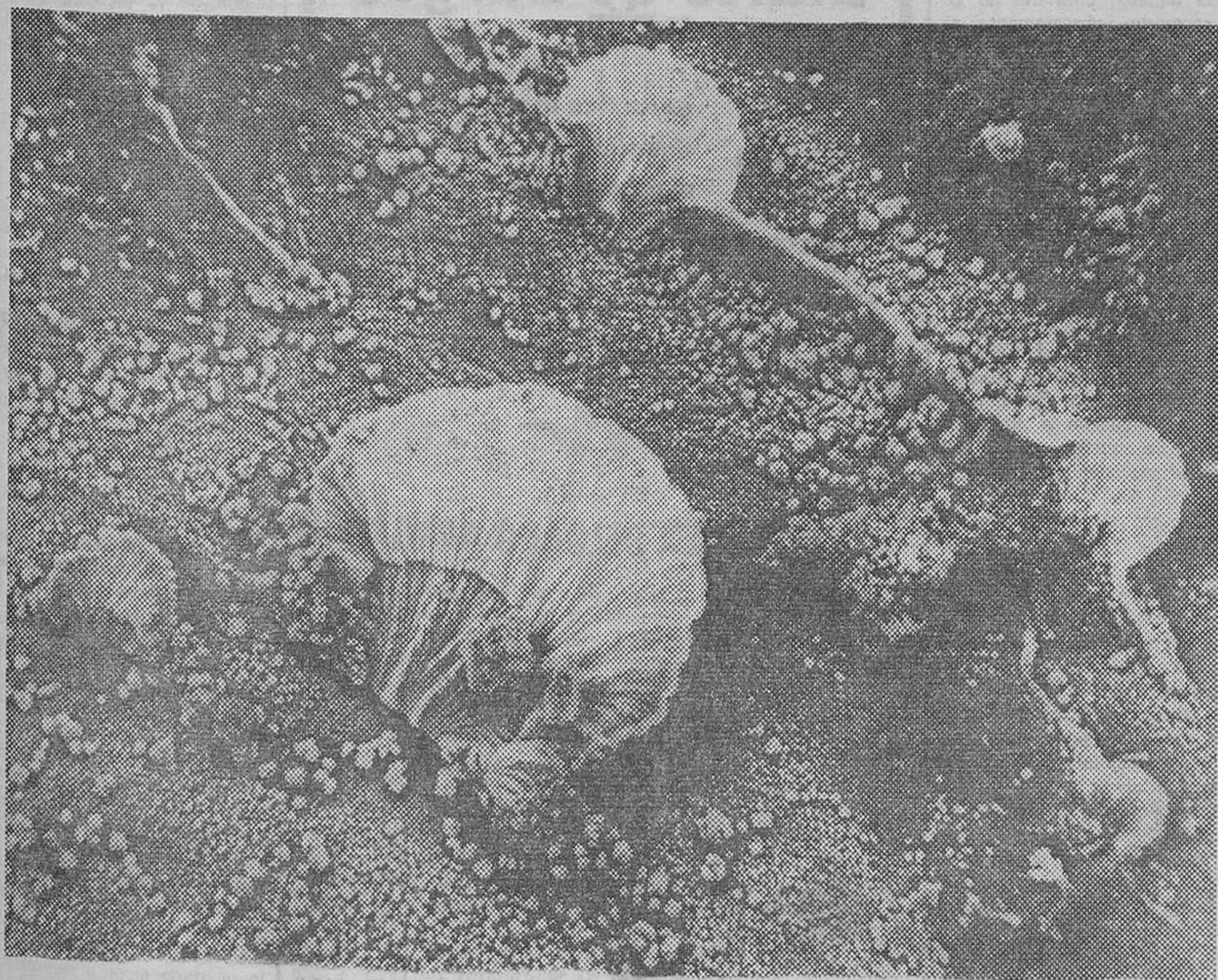
¿Un fondo marino? No. Se trata de una foto realizada gracias a la ayuda del microscopio. En realidad es un colector de corriente de níquel y las conchas son pequeñas aglomeraciones de compuestos cádmicos, que se forman en la fabricación de pilas de gran duración. — (Foto FIEL)
