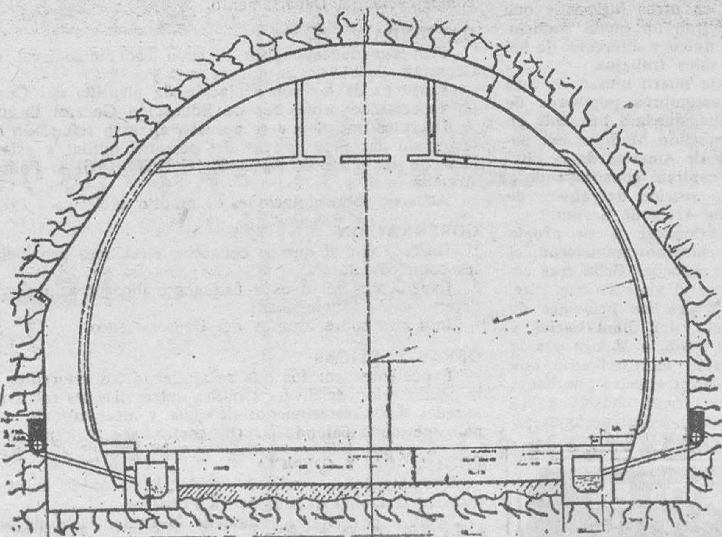
Esta es la sección de la boca del túnel que será construido en el puerto del Escudo. (Foto HOJAS)
