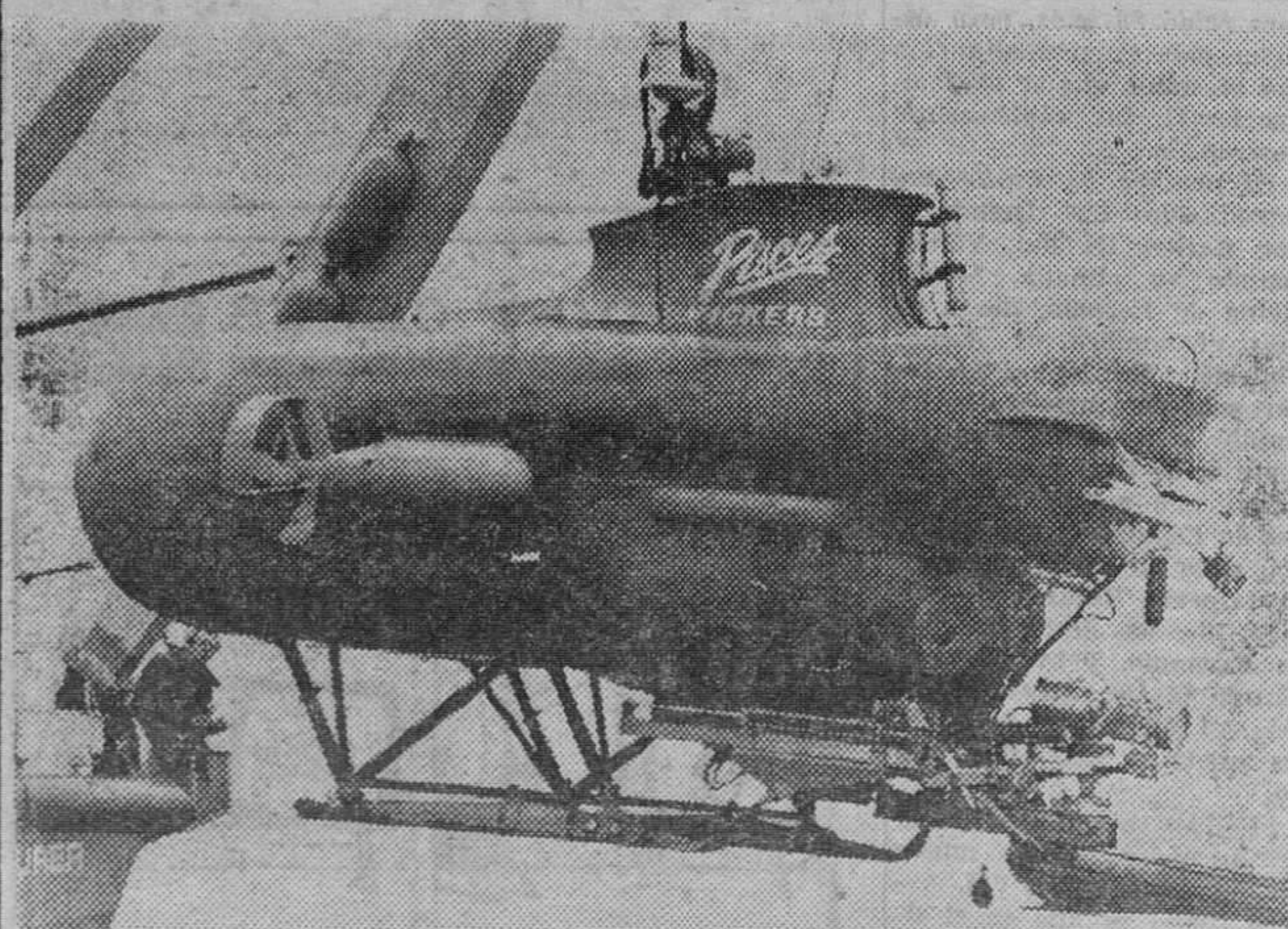
Este es el submarino «Piscis», fabricado por la compañía inglesa Vickers Ltd., que está especialmente diseñado para trabajos de exploración submarina a profundidades de hasta 914 metros. Tiene 6 metros de eslora y una dotación de dos hombres. — (Foto Efe)
