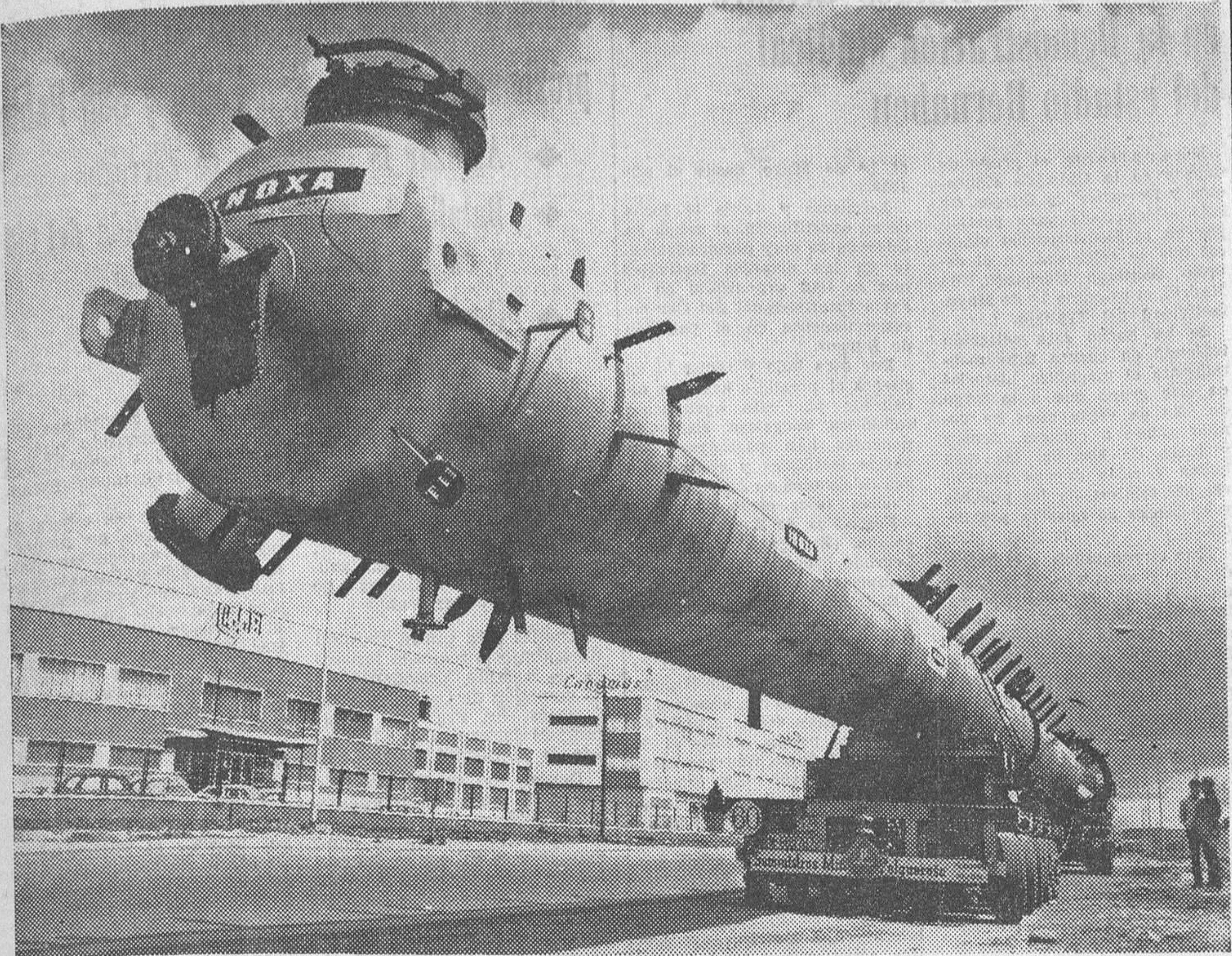
He aquí el transporte que ayer partió de nuestra ciudad, con destino a Tarragona. Se trata de una columna de acero inoxidable, para destilación de butanol y de 36 metros de longitud, fabricada en una importante factoría del "Polo" de Burgos, concretamente "Inoxa". Dicha columna será instalada, como decimos, en el complejo industrial de fertilizantes que en aquella población catalana está montando "Basf Española, S. A.". — (Foto Santi).
