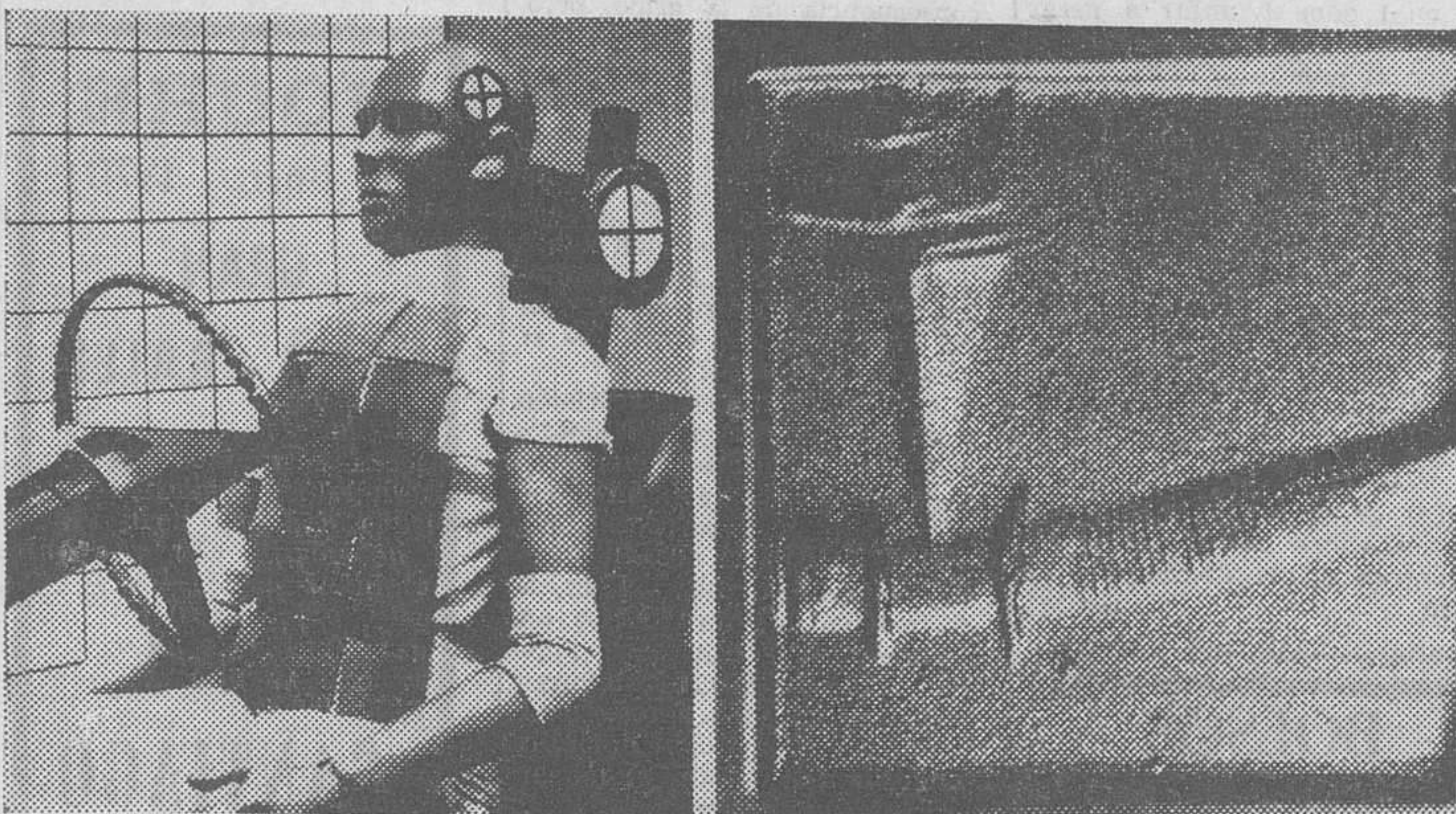
«Metnet» es un nuevo material empleado para medir la presión del volante en un choque simulado. Después de la colisión se ve, a la derecha, cómo se han marcado las huellas del volante. (Foto CIFRA)
