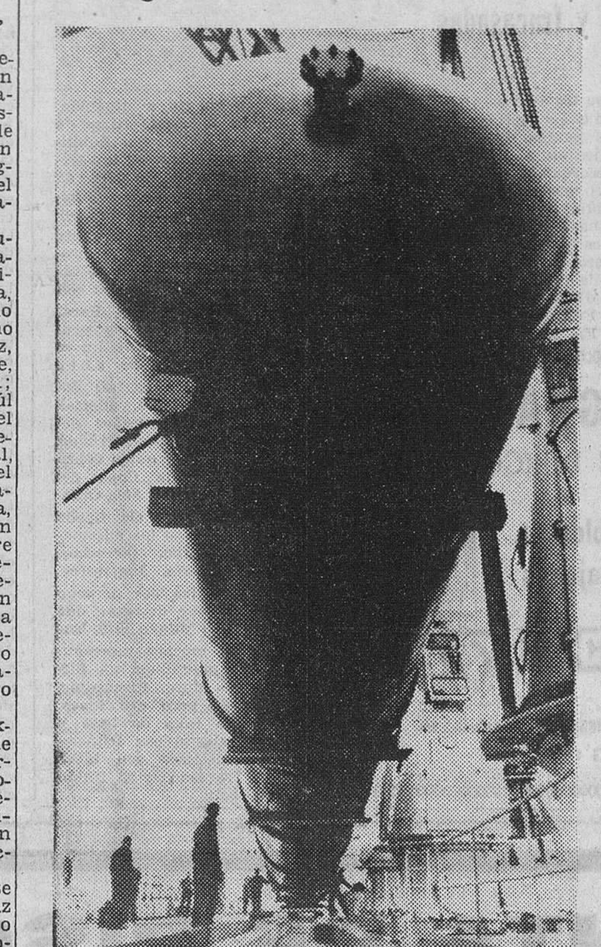
Más de 33 metros de largo y tres de diámetro mide este gigantesco «cigarro» de 60 toneladas que una enorme grúa instala sobre la cubierta del carguero «Trinidad» en el puerto de Hamburgo. Se trata en realidad de una enorme pieza para la industria química en Filipinas. Tres semanas de viaje tardará en llegar a su destino. — (Foto FIEL)
