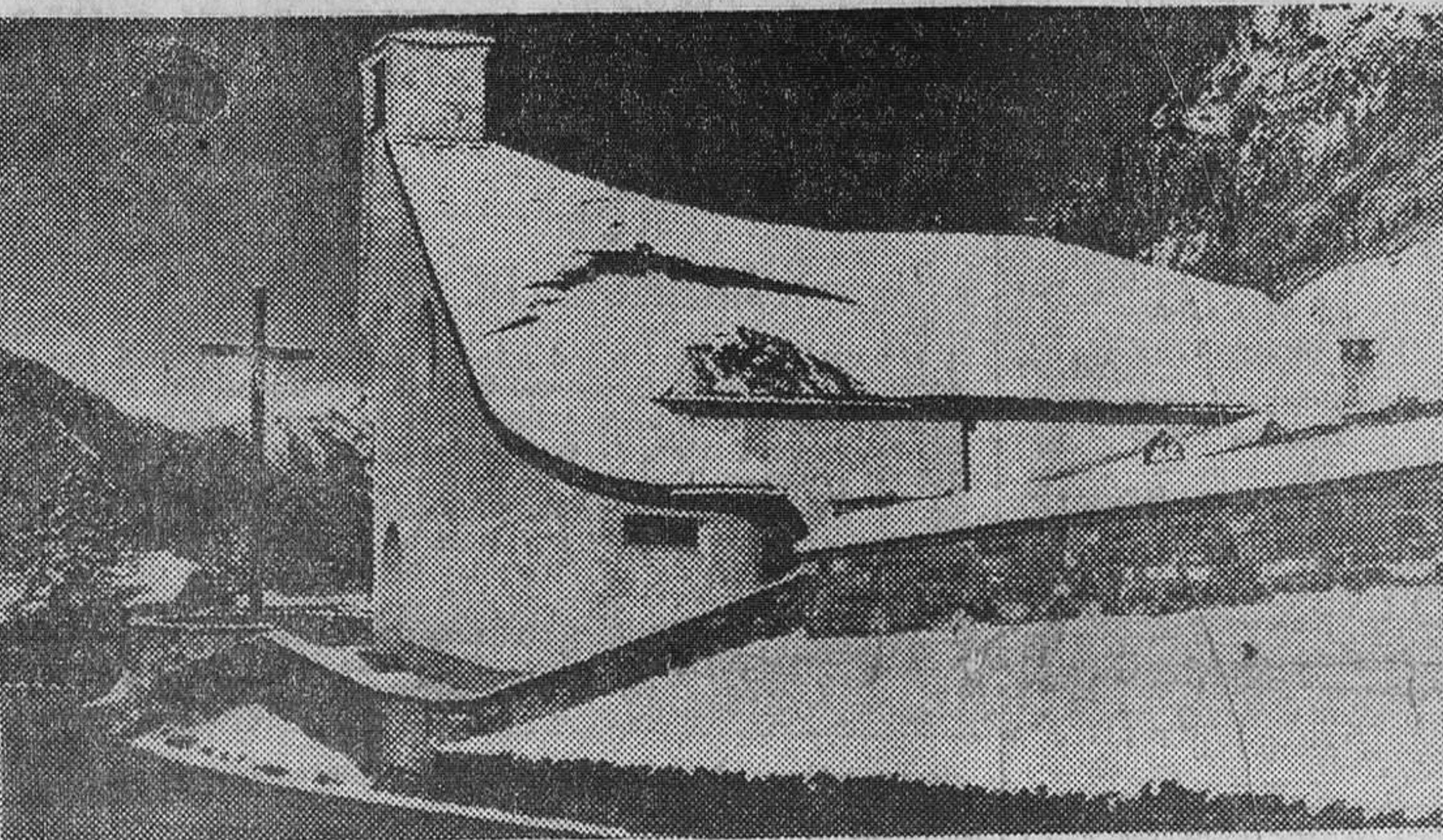
En término de Langen, en el Arlberg alemán, se ha construido esta iglesia especialmente diseñada para evitar los peligros de los aludes de hielo y nieve en el invierno. Se trata de una especie de «bunker» y cuya parte que da a la montaña tiene forma de tres esquinas, de modo que en caso de alud lo corte y lo haga rebasar el edificio. La entrada está bajo la torre. Si el modelo resulta eficaz se construirán otras iglesias como esta en Suiza y Austria. — (Foto FIEL)
