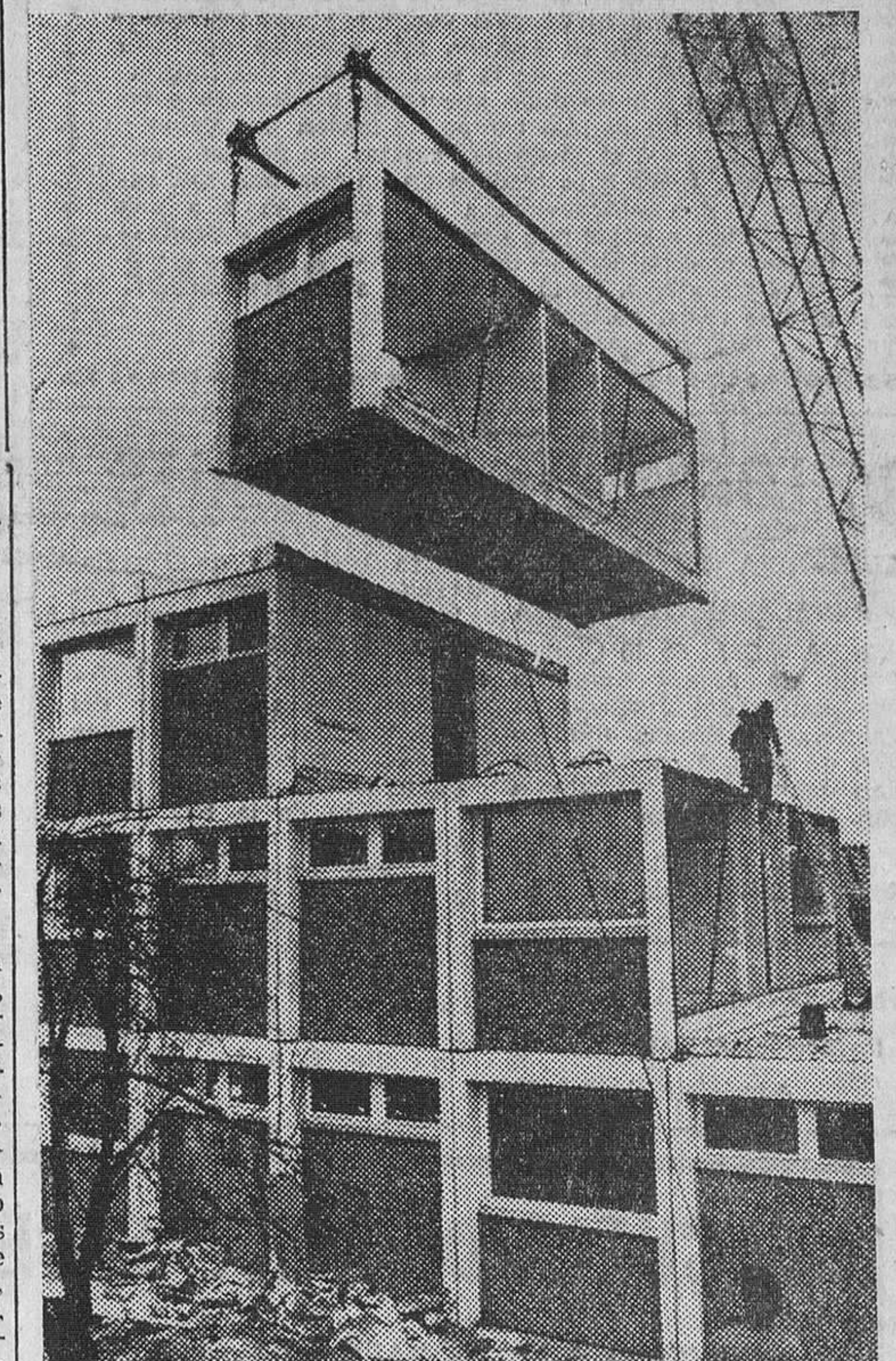
En tan sólo ocho horas puede estar terminada una casa de viviendas de tres pisos según el proyecto que está llevando ahora a la práctica la firma alemana Variel de Buxtehuder. El sistema es, naturalmente, a base de elementos prefabricados. Una gigantesca grúa de 125 toneladas coloca el conjunto de 24 elementos con sus correspondientes escaleras en el plazo de veinte minutos, tal como vemos en esta fotografía. Además, al hacerse en serie estos módulos o piezas, el costo se abarata en gran parte. He aquí, pues, una solución para el urgente problema de la vivienda que tienen planteado numerosas ciudades. — (Foto FIEL)
