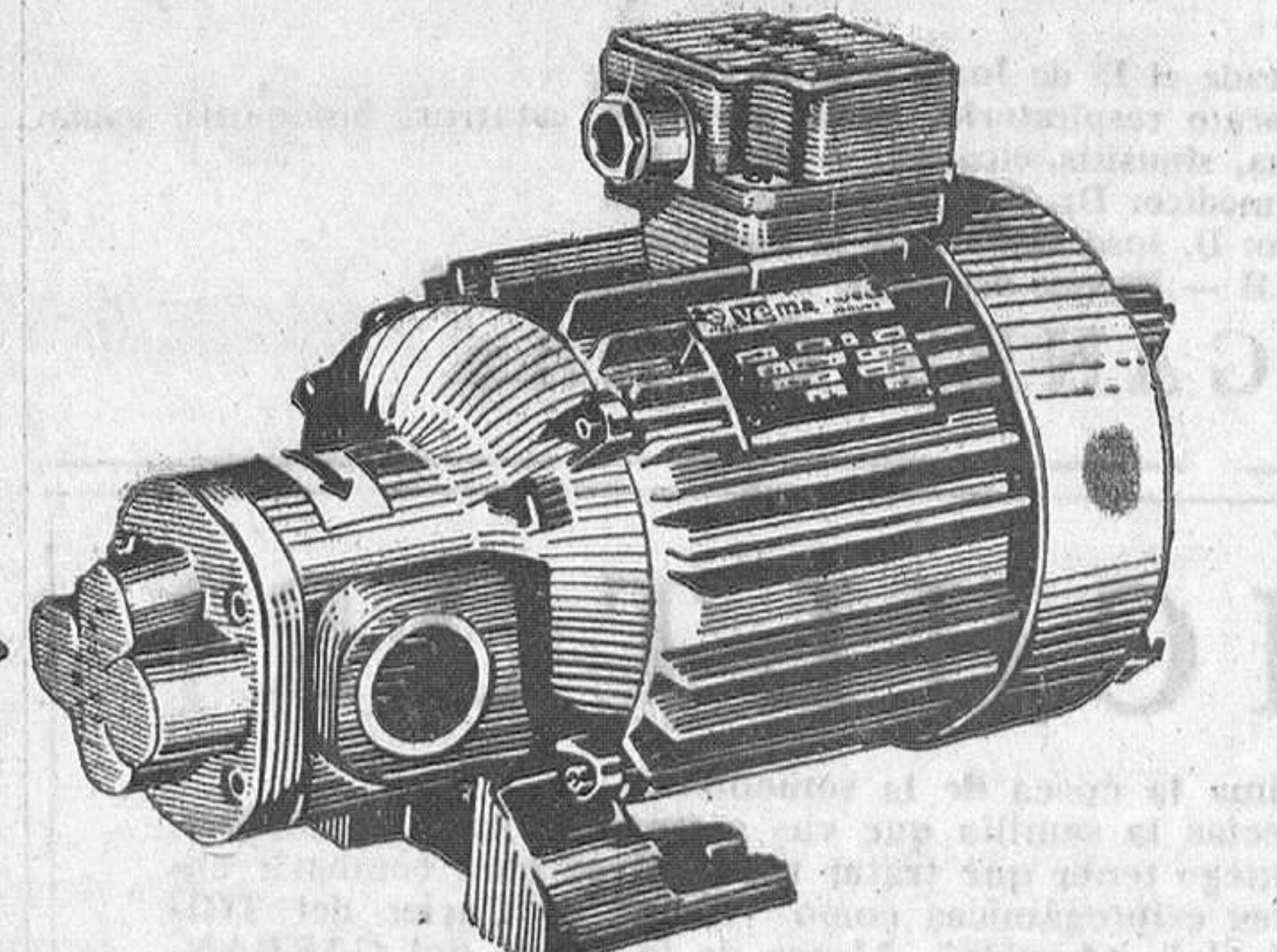
«Tipo NFT 61/7» C. V. 0,30 - Trif. Caudal: de 320 a 255 Kgs h. Altura: de 10 a 60 metros.
