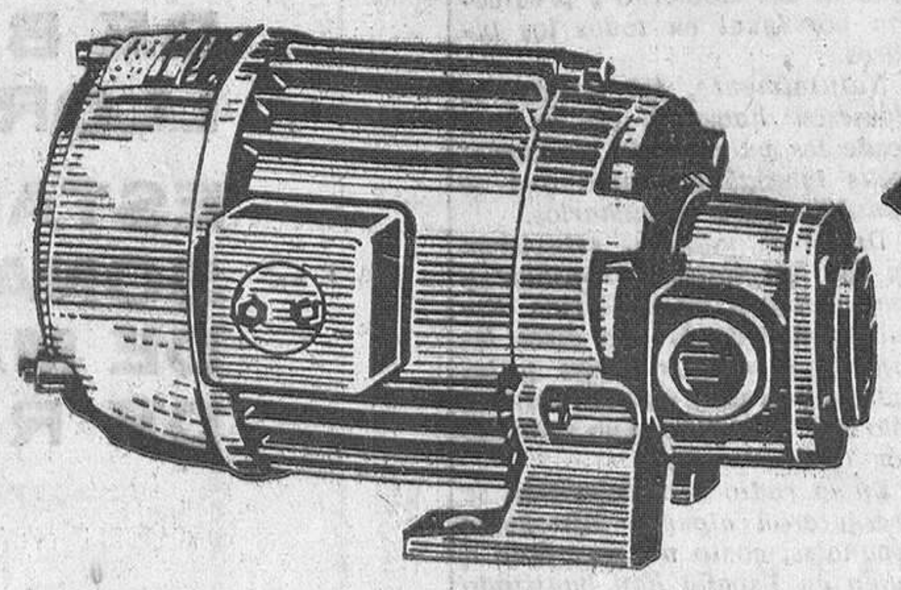
«Tipo NFT 61/7» C. V. 0,30 - Trif. Caudal: de 320 a 255 Kgs h. Altura: de 10 a 60 metros.
