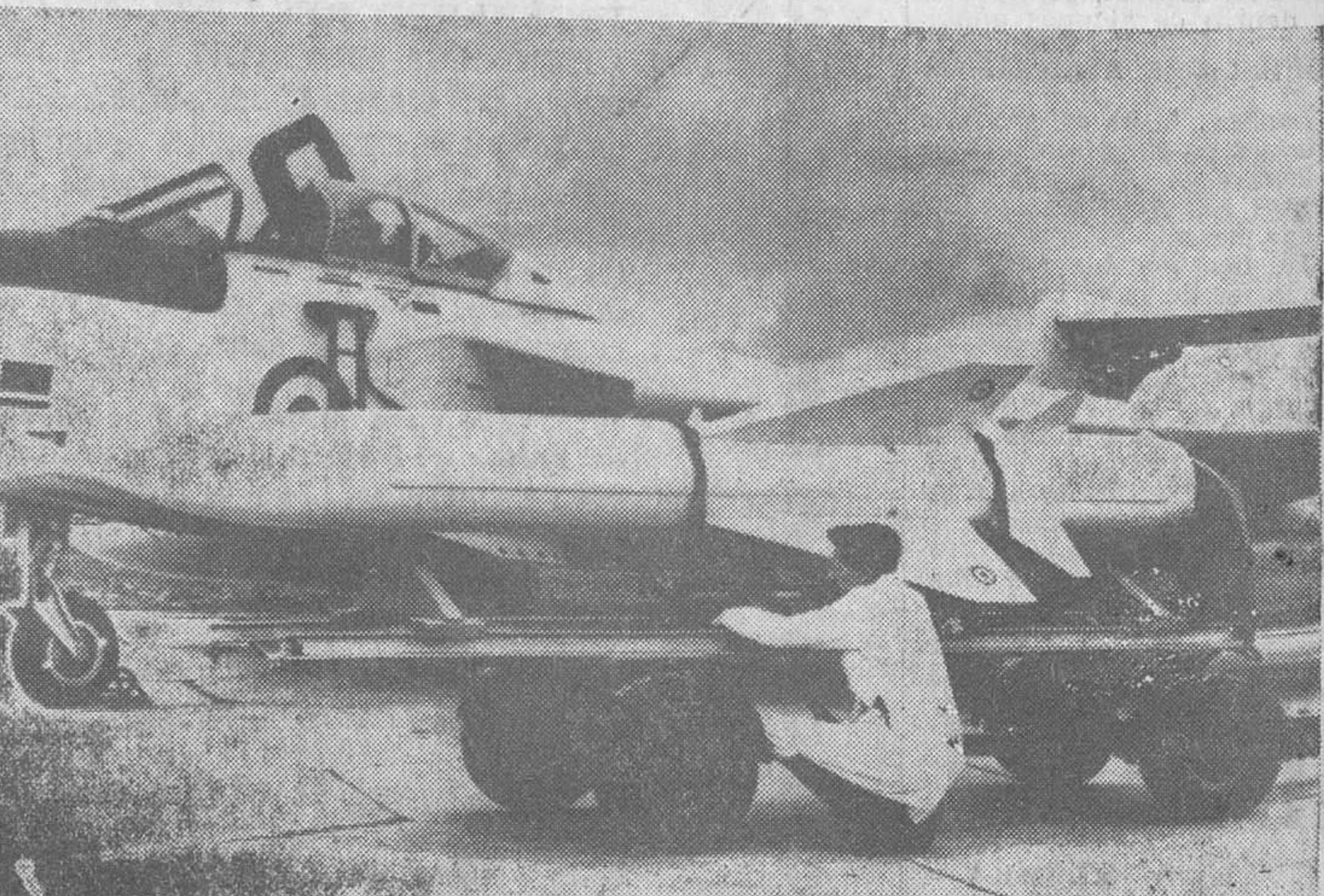
Esta es la primera fotografía obtenida del misil «Martel», cohete aire-tierra de precisión táctica, que ha sido diseñado y construido conjuntamente por Inglaterra y Francia. El «Martel», (misil anti-radar y televisión), ha sido creado para abastecer las Fuerzas Armadas de ambos países. (Foto Fiel)
