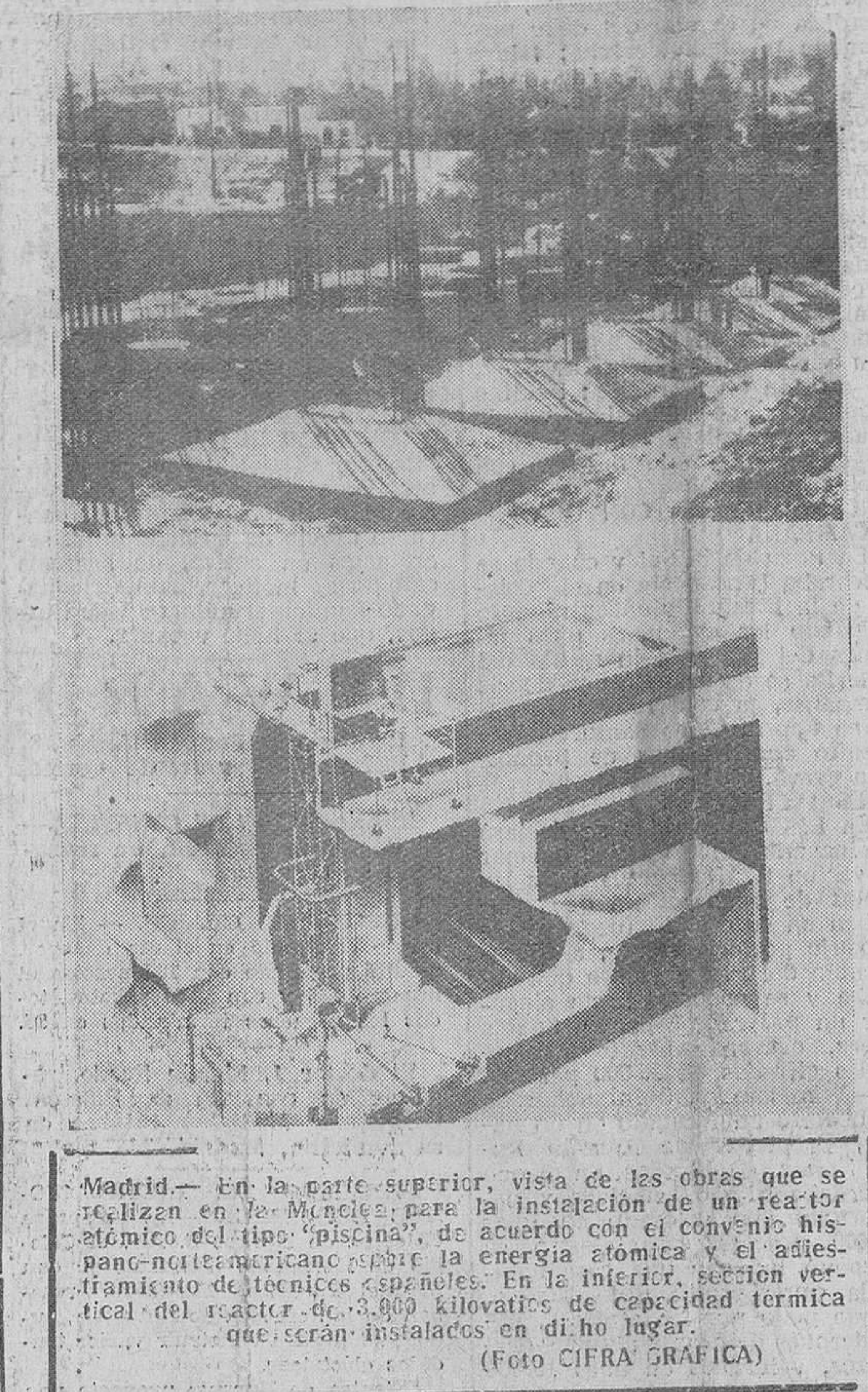
Madrid.— En la parte superior, vista de las obras que se realizan en la zona de la instalación de un reactor atómico del tipo “piscina”, de acuerdo con el convenio hispano-norteamericano sobre la energía atómica y el adiestramiento de técnicos españoles. En la inferior, sección vertical del reactor de 3.000 kilovatios de capacidad térmica que serán instalados en dicho lugar. (Foto CIFRA GRAFICA)
