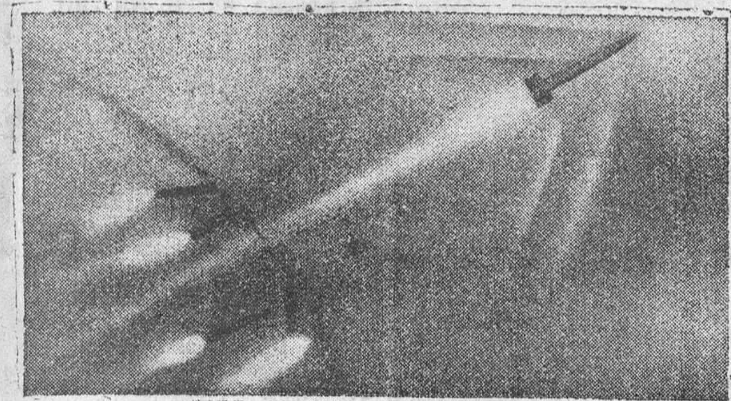
El tubo. El aire así comprimido se mezcla con el combustible encendido y los gases resultantes de esta combustión salen por la parte trasera del tubo propulsándolo hacia adelante. Para lanzar el autorractor se preciso utilizar otra forma de energía, tal como cohetes. — (Foto C.)
