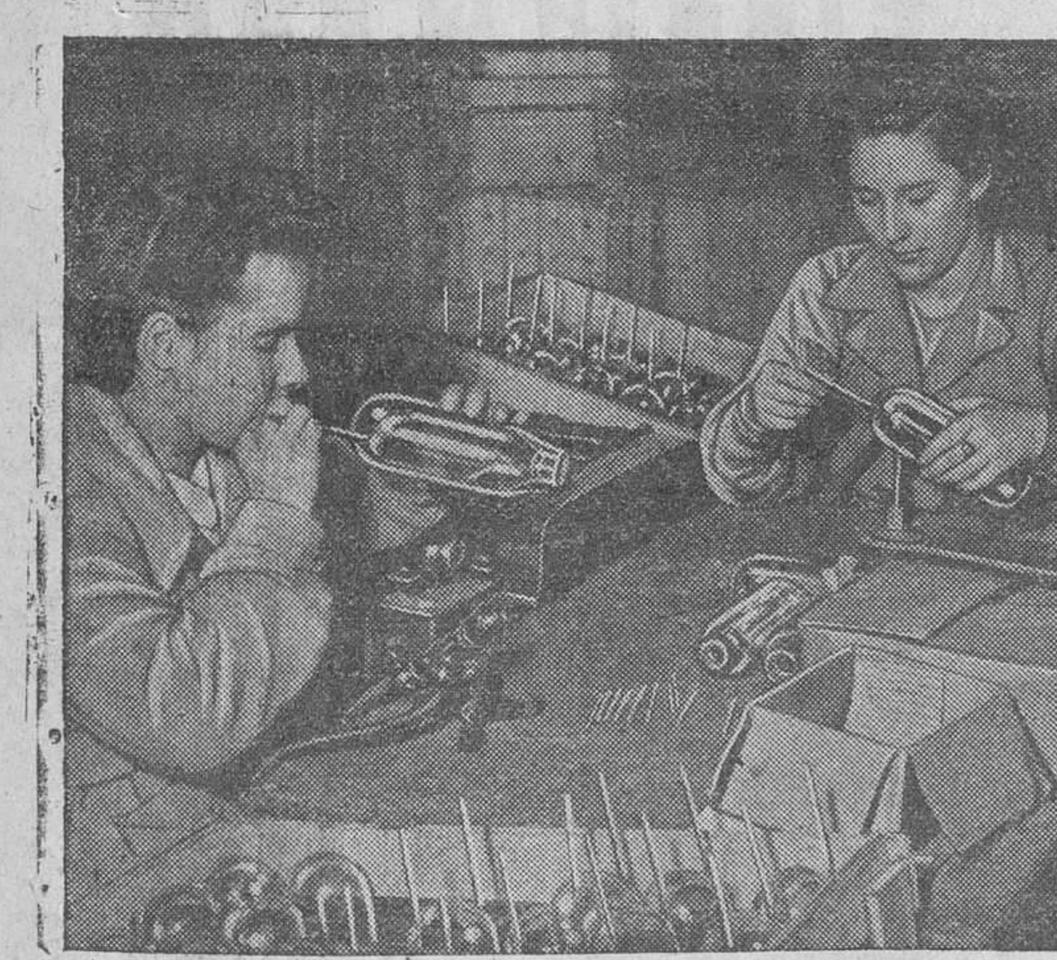
La producción de termos en la Gran Bretaña alcanza la cifra de 70.000 por semana. Estas operarias aplican la varilla de cristal que permite plantear y realizar la operación de vaciado del termo. (Foto Calpe)
