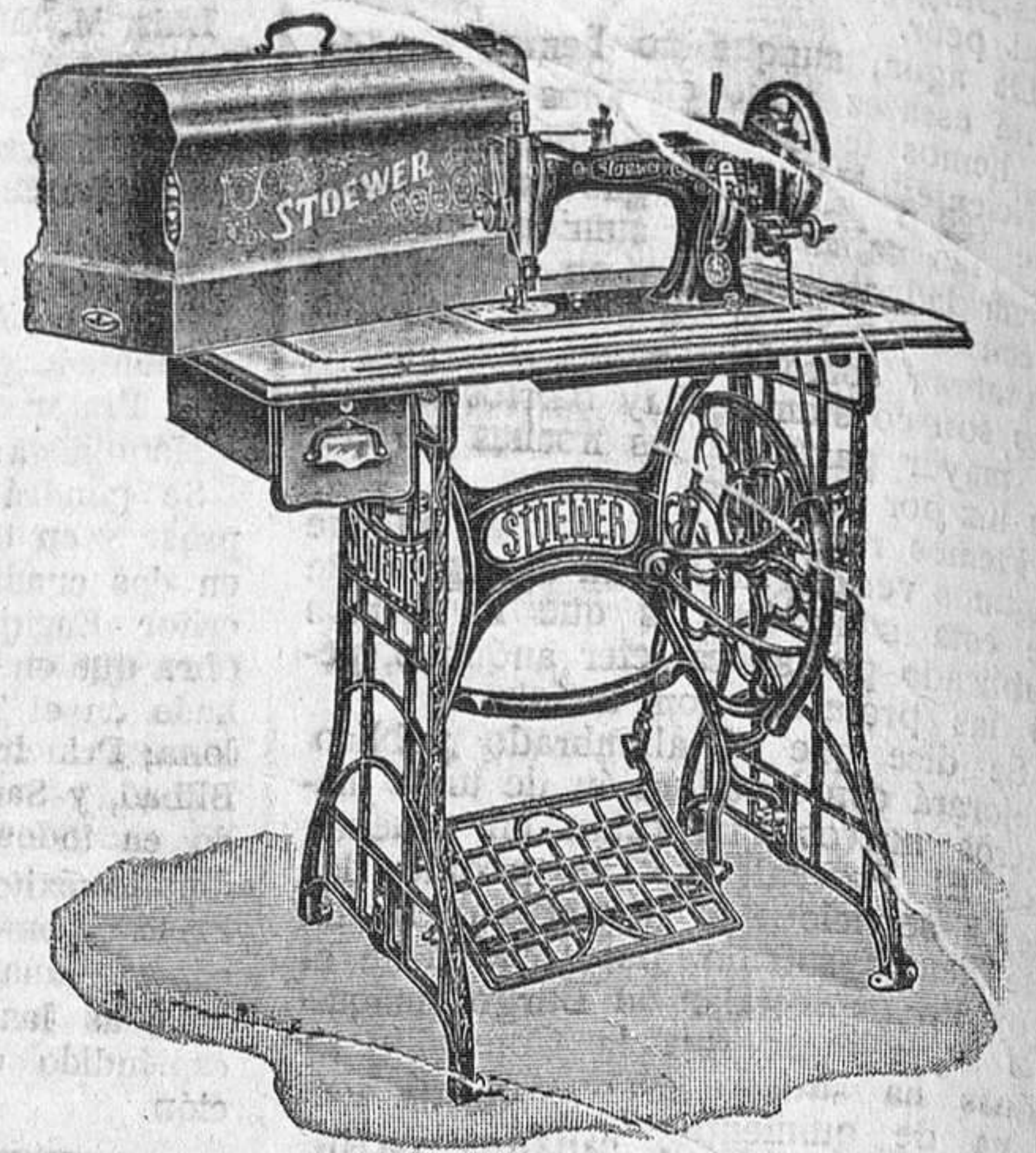
Máquina familiar, cose hacia adelante y hacia atrás, rozamiento sobre bolas, 280 pesetas.
