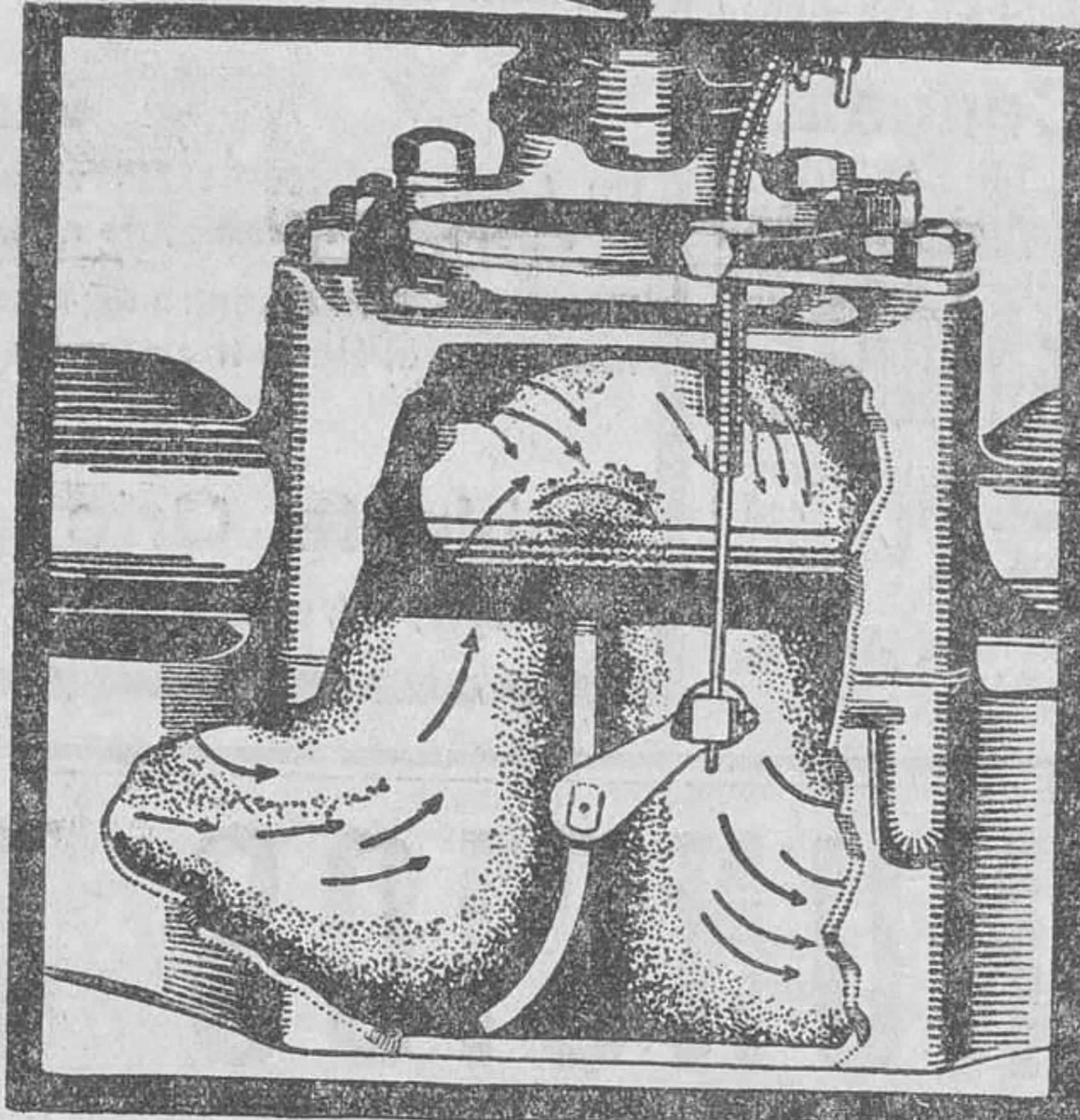
El regulador del calor de la mezcla facilita el rápido calentamiento del motor, asegurando mejor rendimiento en verano y en invierno.
