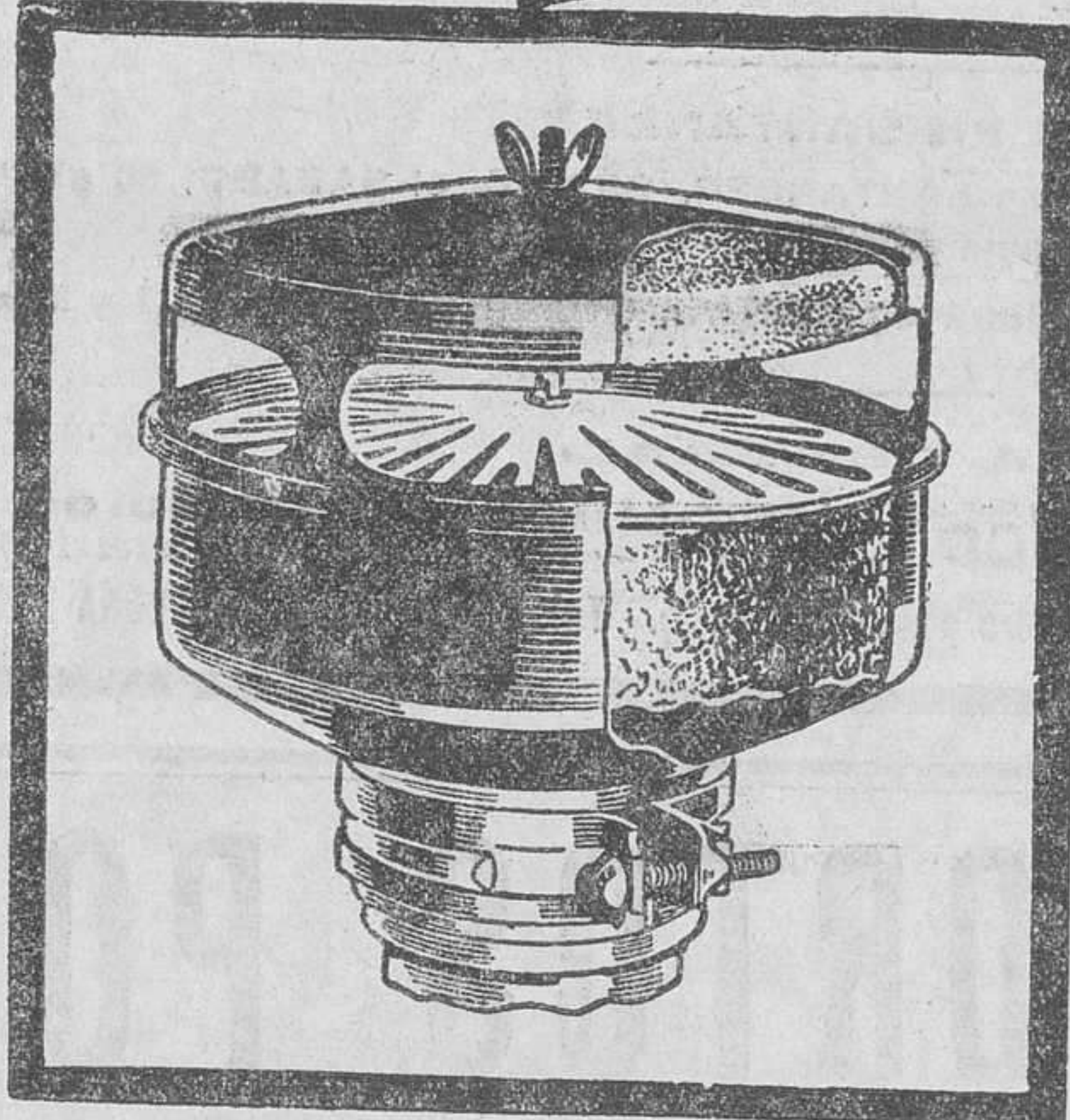
El purificador de aire evita la entrada de polvo y otras materias extrañas que impiden el buen funcionamiento del motor y causan extraordinario desgaste.
