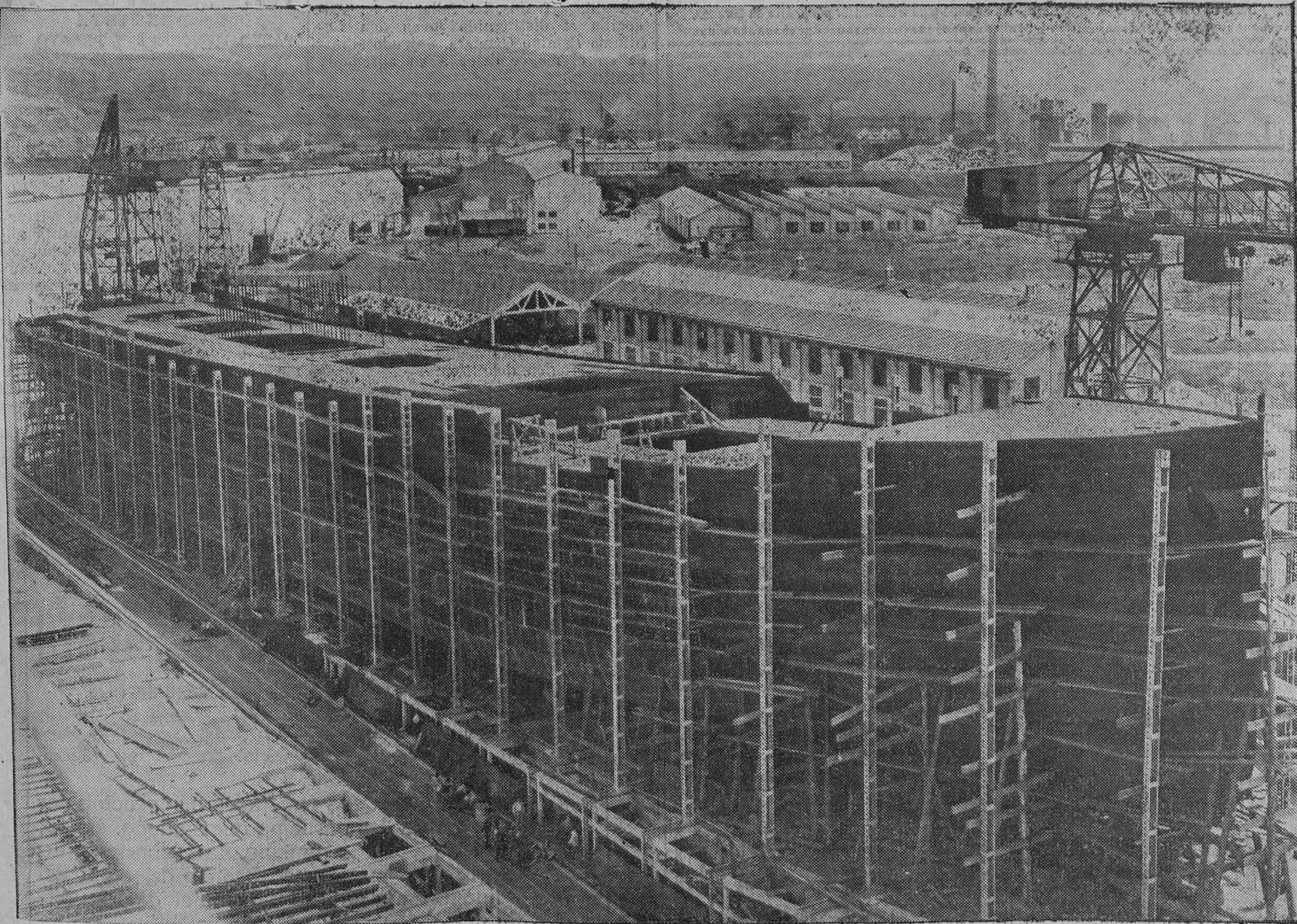
EL CABO SAN ANTONIO, en construcción en los Astilleros de la Constructora Naval, en Sestao, para la Empresa naviera IBARRA Y COMPAÑIA, con destino a la línea Mediterráneo-Brasil-Plata. Propulsado por motores Diesel. Eslora total, 152 metros. Manga, 19'28 metros. Puntal, 11'28 metros. Desplazamiento, 16.500 toneladas. Velocidad, 17 1/2 millas.
