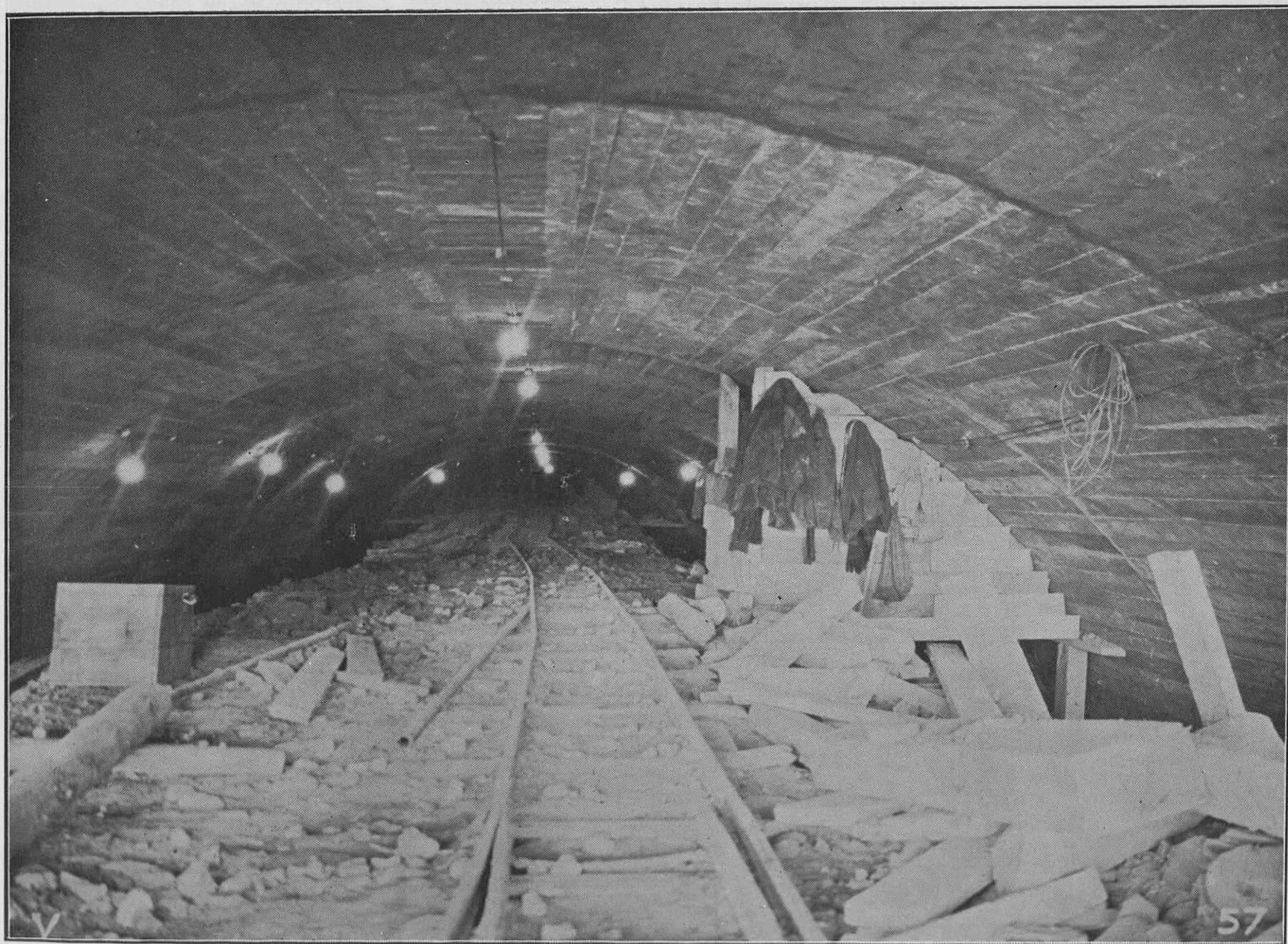
Interior del primer túnel que se construye para el nuevo ferrocarril Santander-Mediterráneo.
