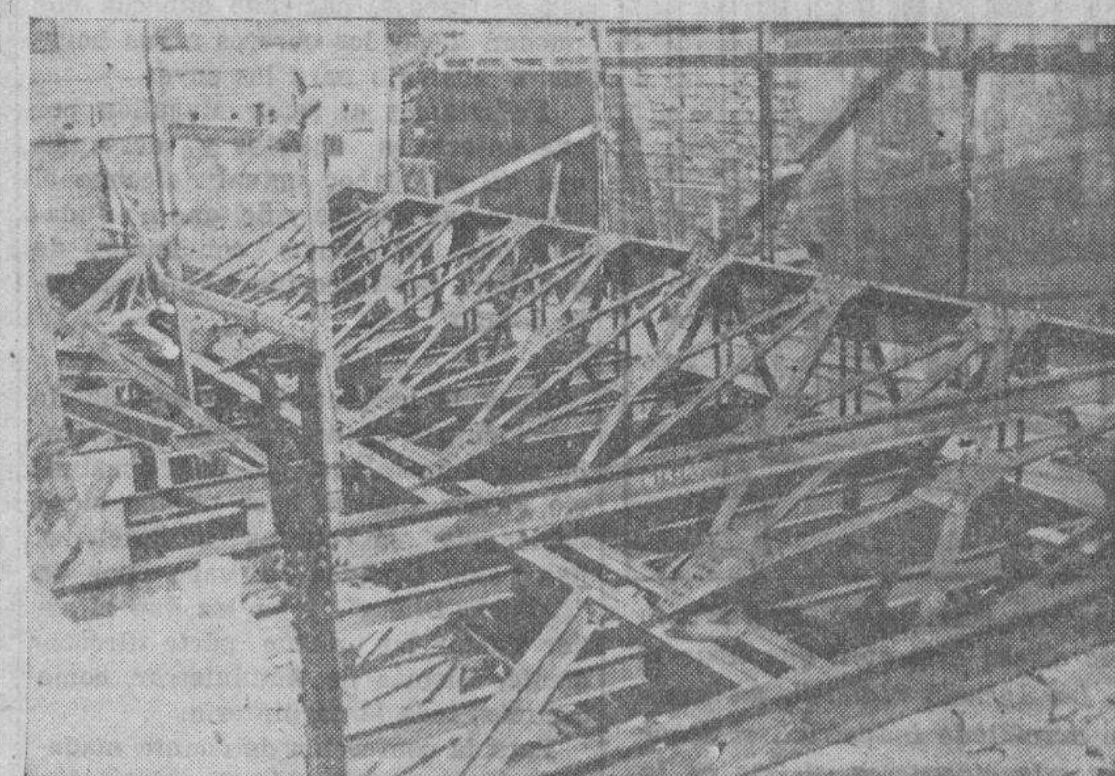
Estructura metálica construída en los "Talleres Zaragoza", de don José González Torres (antigua Casa "Zaragoza-Industrial").
