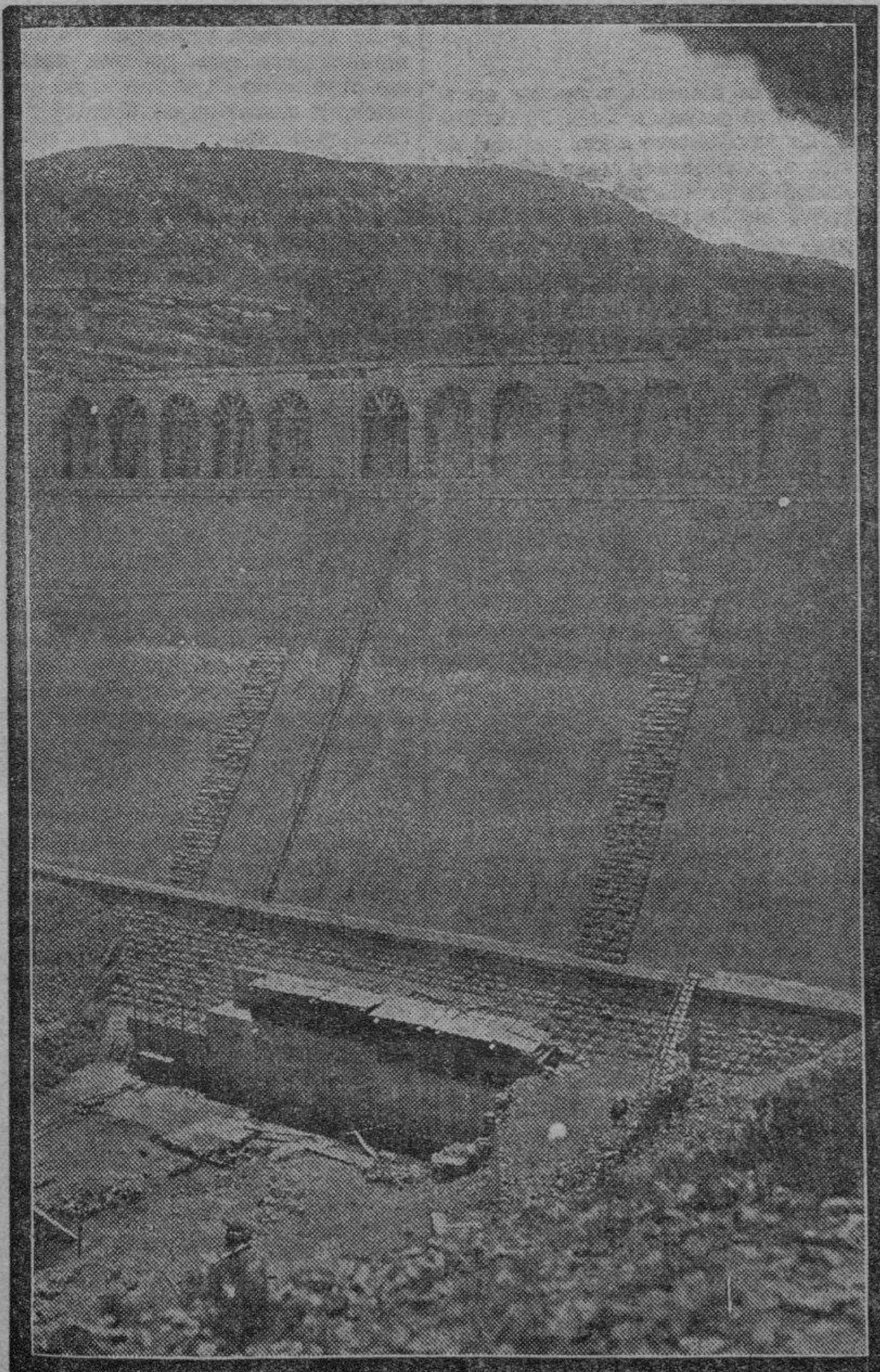
Muro de contención del Pantano que ha de dar vida a la comarca bajoaragonesa.
