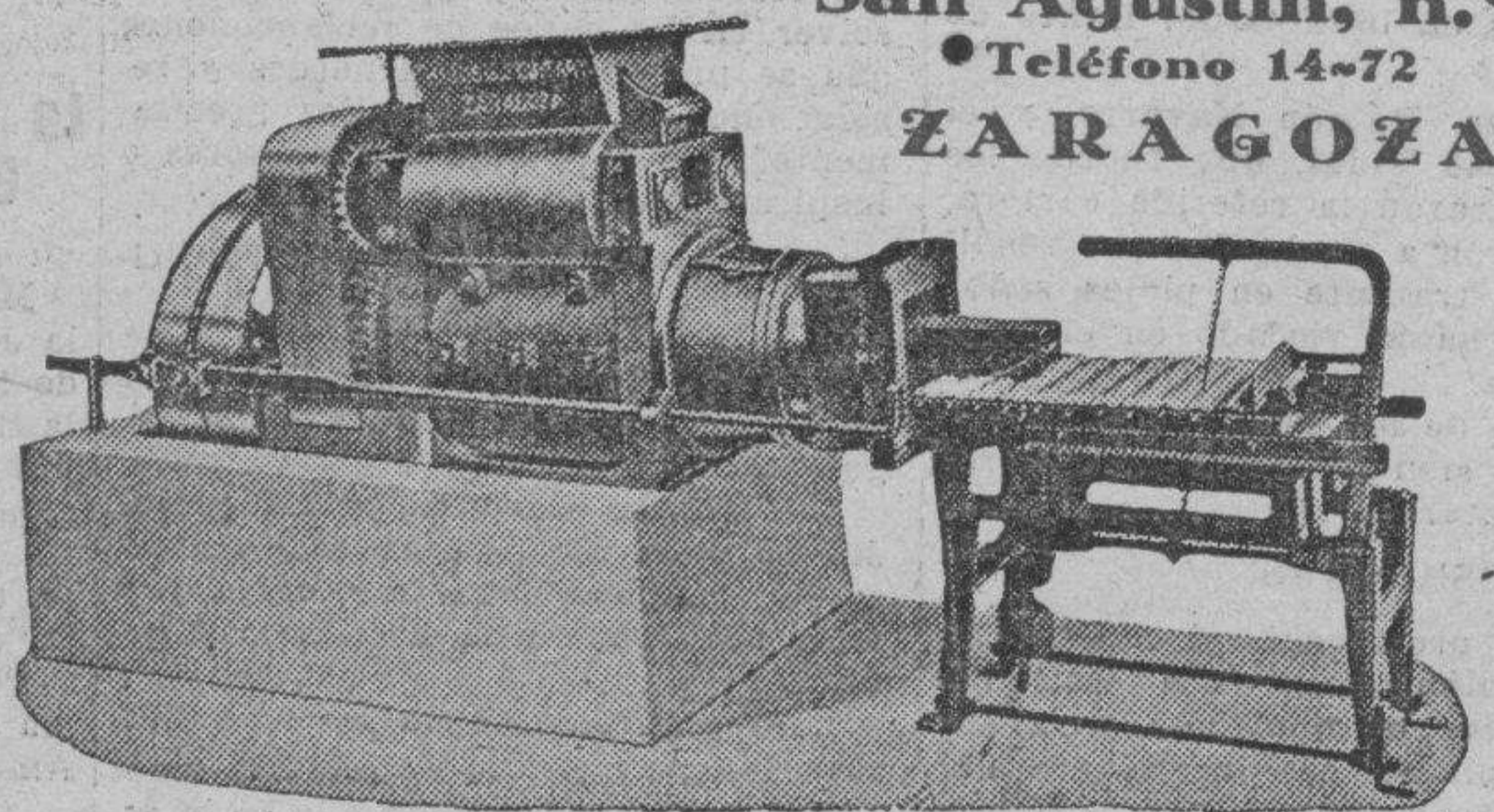
Galletera para ladrillo hueco, macizo, etc., etc.
