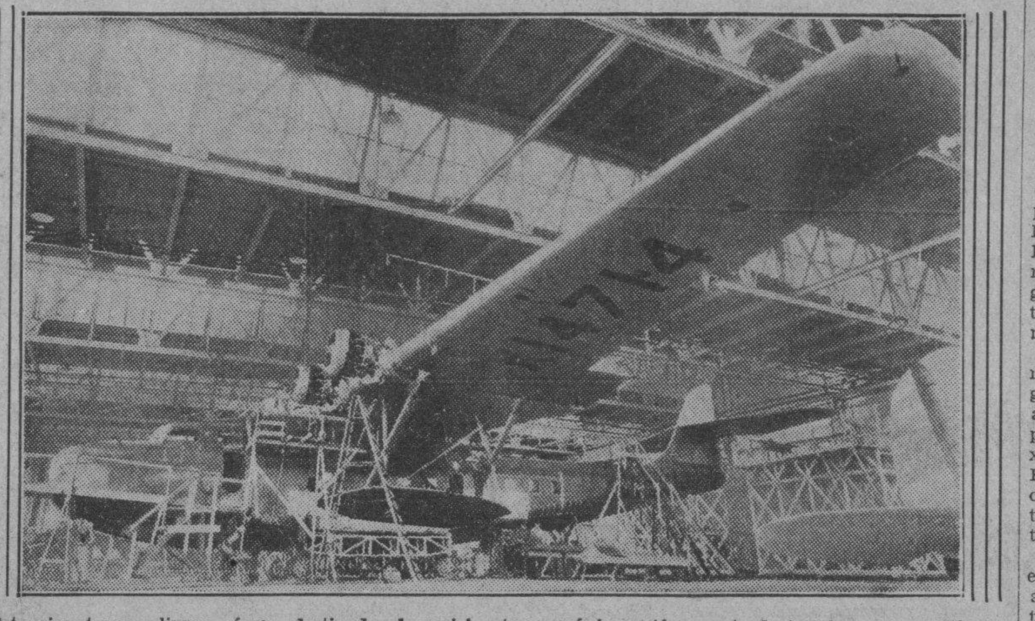
Este gigantesca «clipper aéreo», destinado al servicio transoceánico, está a punto de terminarse en Baltimore, donde ha estado en construcción durante dos años, lejos de las miradas de los curiosos. Fue ordenado por la Pan American, empresa que sostiene que dicho aparato podrá transportar 50 pasajeros sobre el Atlántico o el Pacífico a una velocidad de tres millas por minuto.
