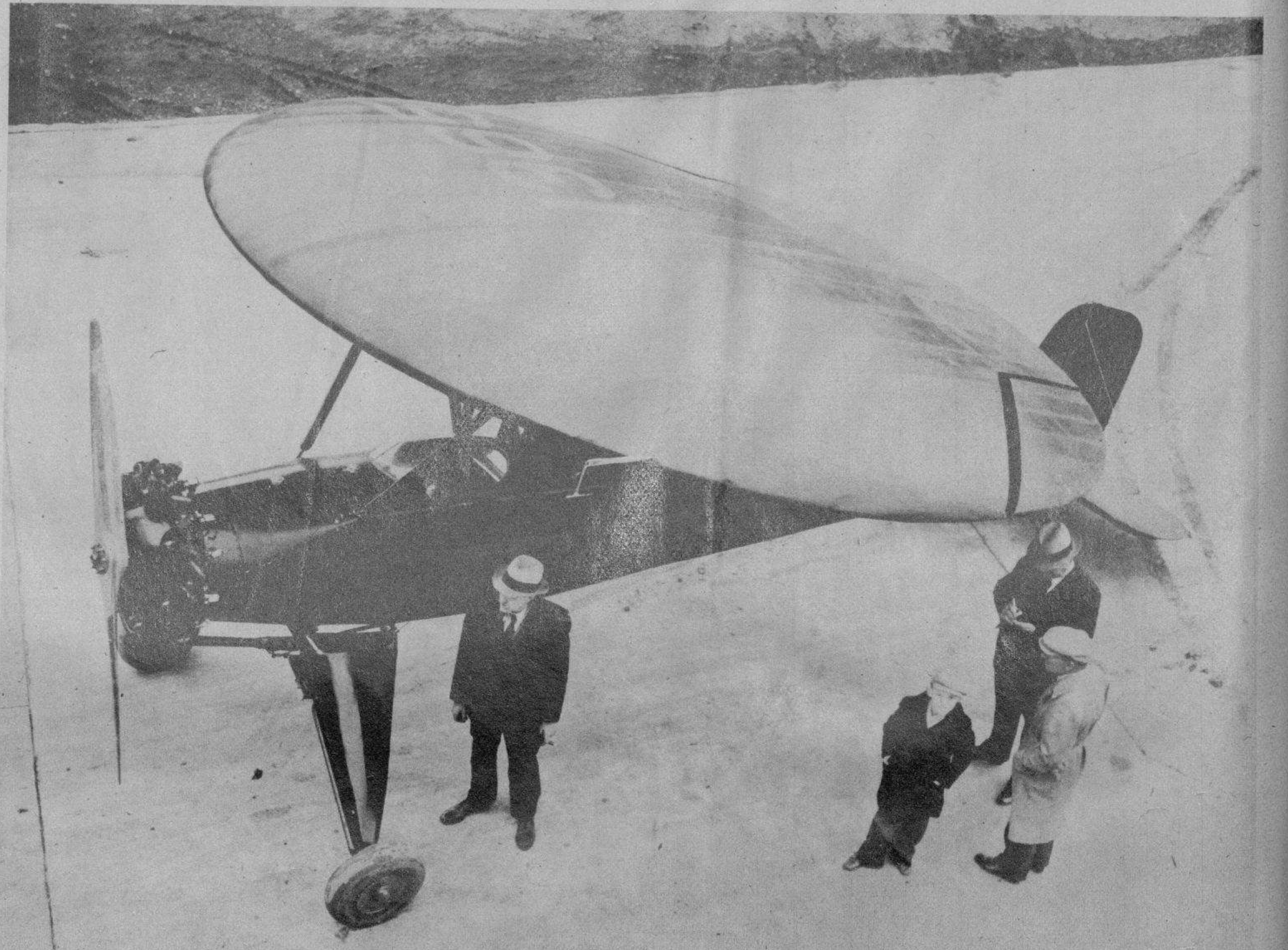
NUOVO AEROPLANO: EL CIRCOPLANO. —Se llama este aparato curioso el "circoplano", inventado por los ingenieros mecánicos Mr. Ray Stein y C. Burkland Hart. Este aparato tiene un ala circular en forma de paraguas o paracaídas y es capaz de aterrizar tomando un ángulo de sesenta grados en un área de veinticinco
