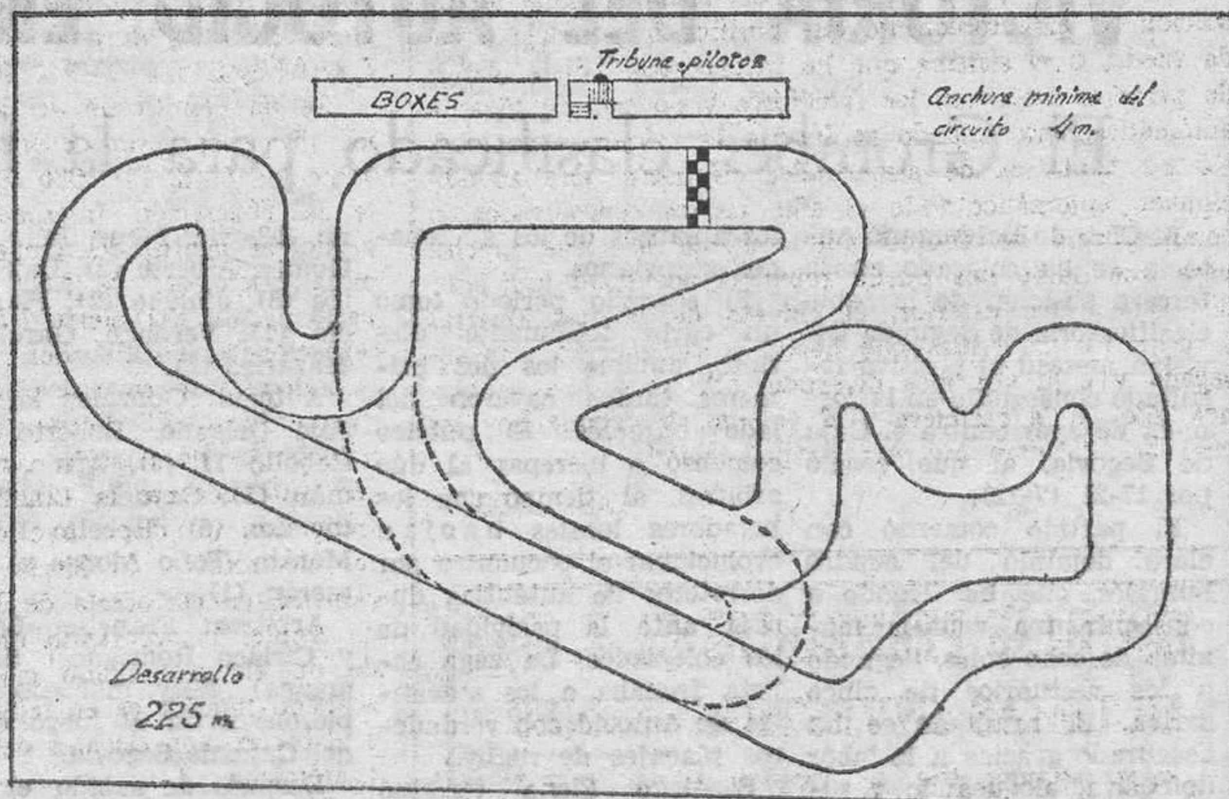
Plano del circuito permanente que se construirá en las cercanías de San Isidro donde se albergarán las pruebas competitivas de Automodelismo «Todo Terreno».
