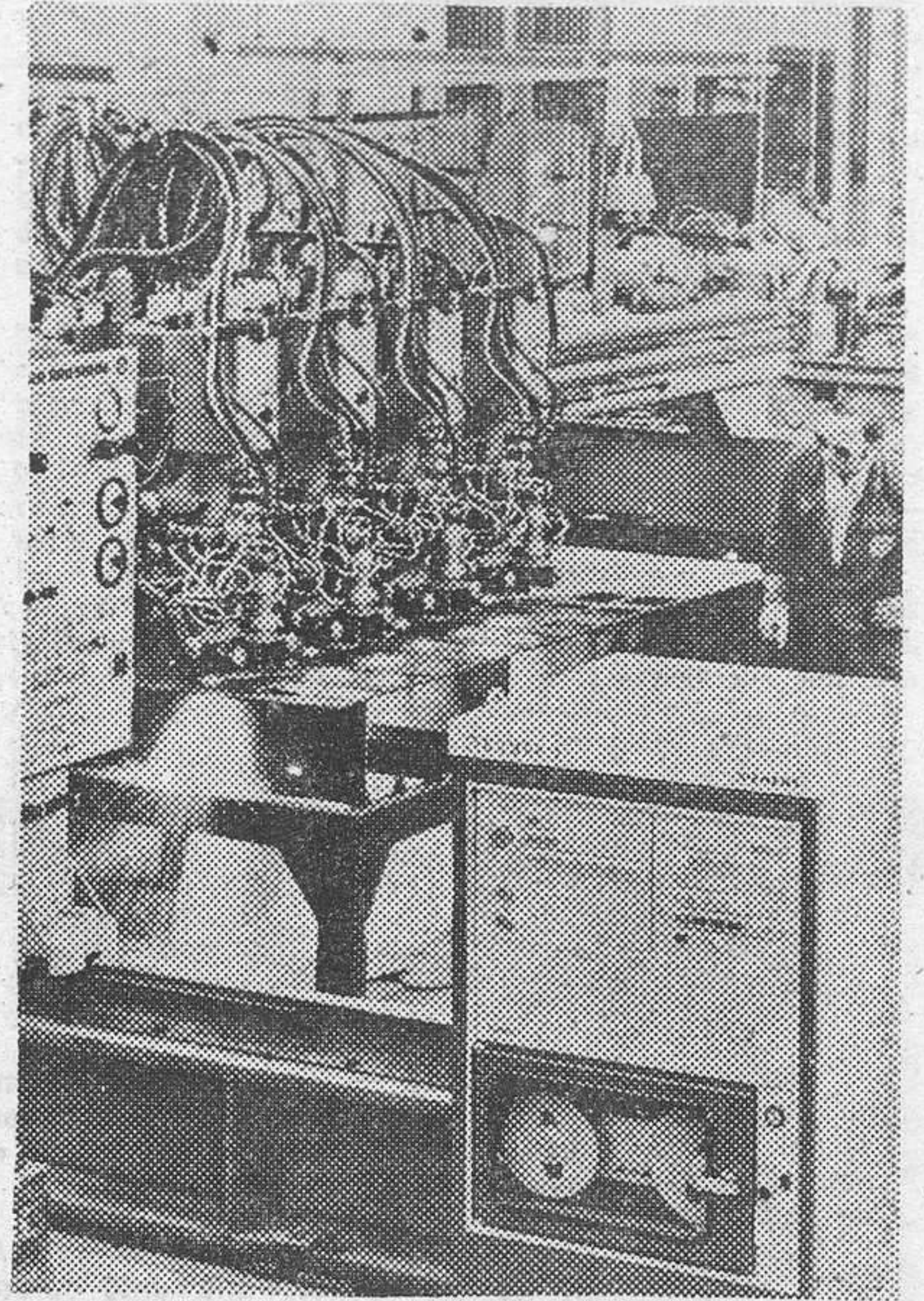
El nivel industrial y tecnológico de Alemania Occidental se eleva constantemente y permite la producción de material altamente perfeccionado, como este mando numérico de controlado por microprocesador para máquinas de oxígeno creados por Siemens. — (Foto EFE-FIEL)
