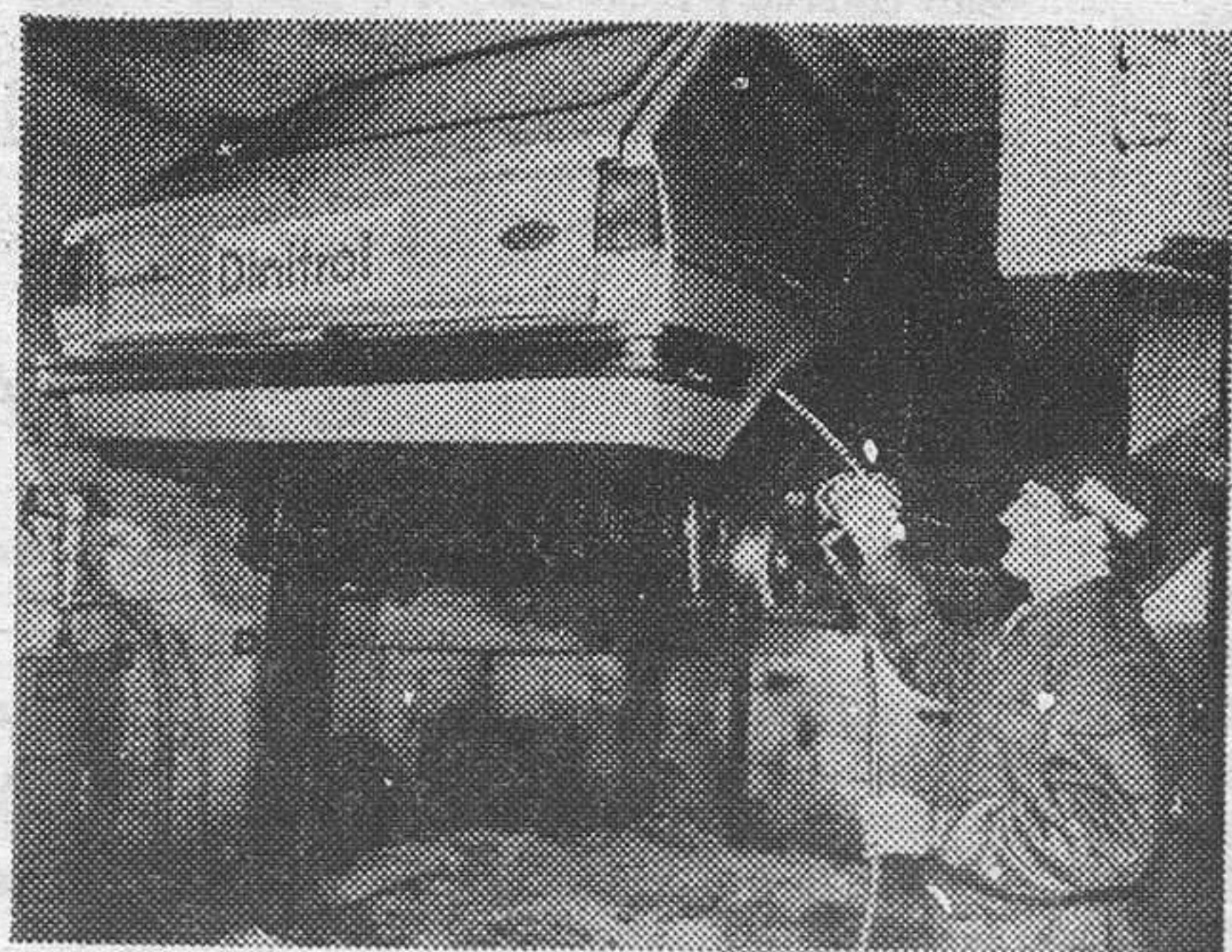
Pulverización del DINITROL Metalic en el pasárreudas
