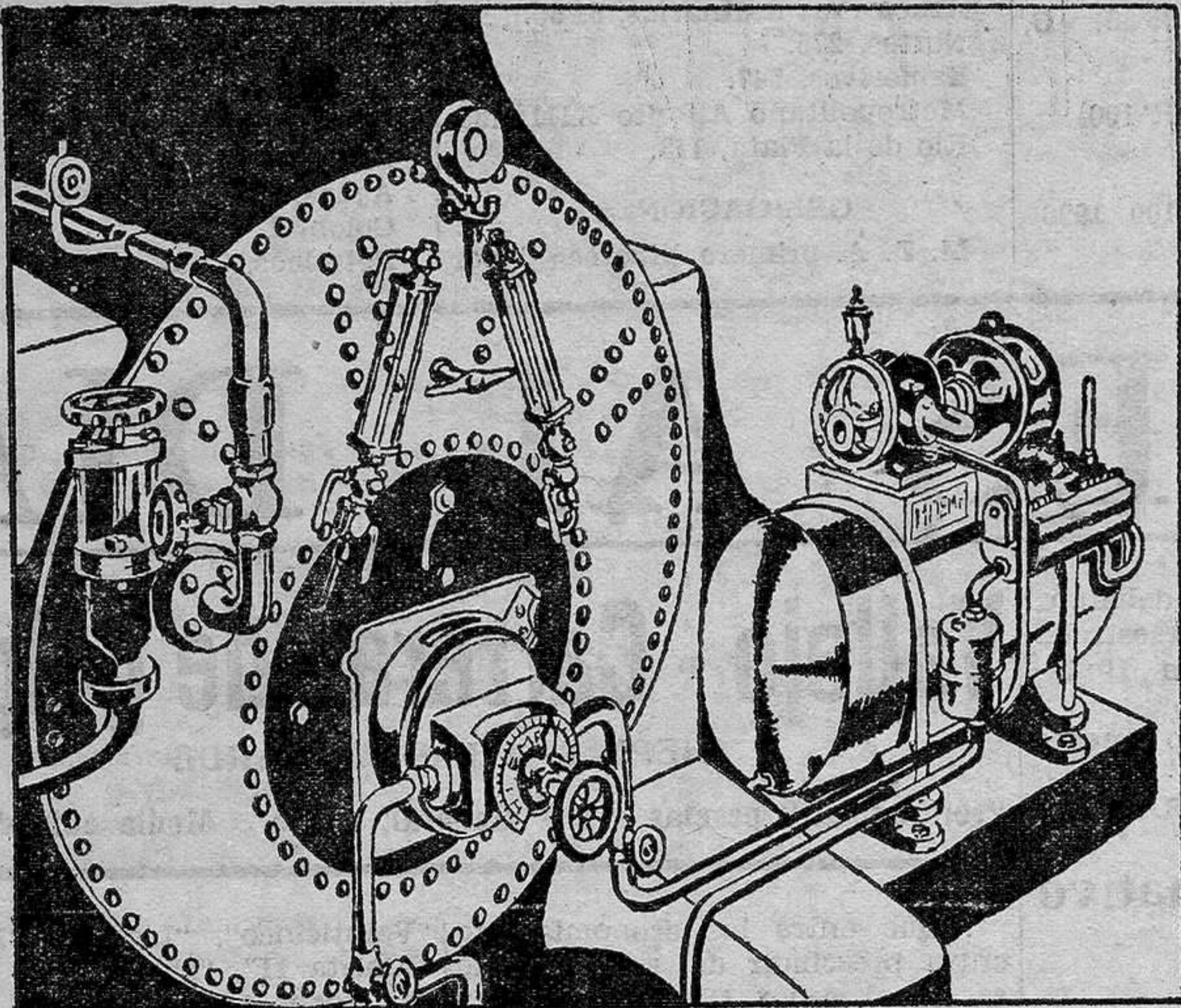
GRUPO «HDEME» APLICADO A UNA CALDERA DE VAPOR
