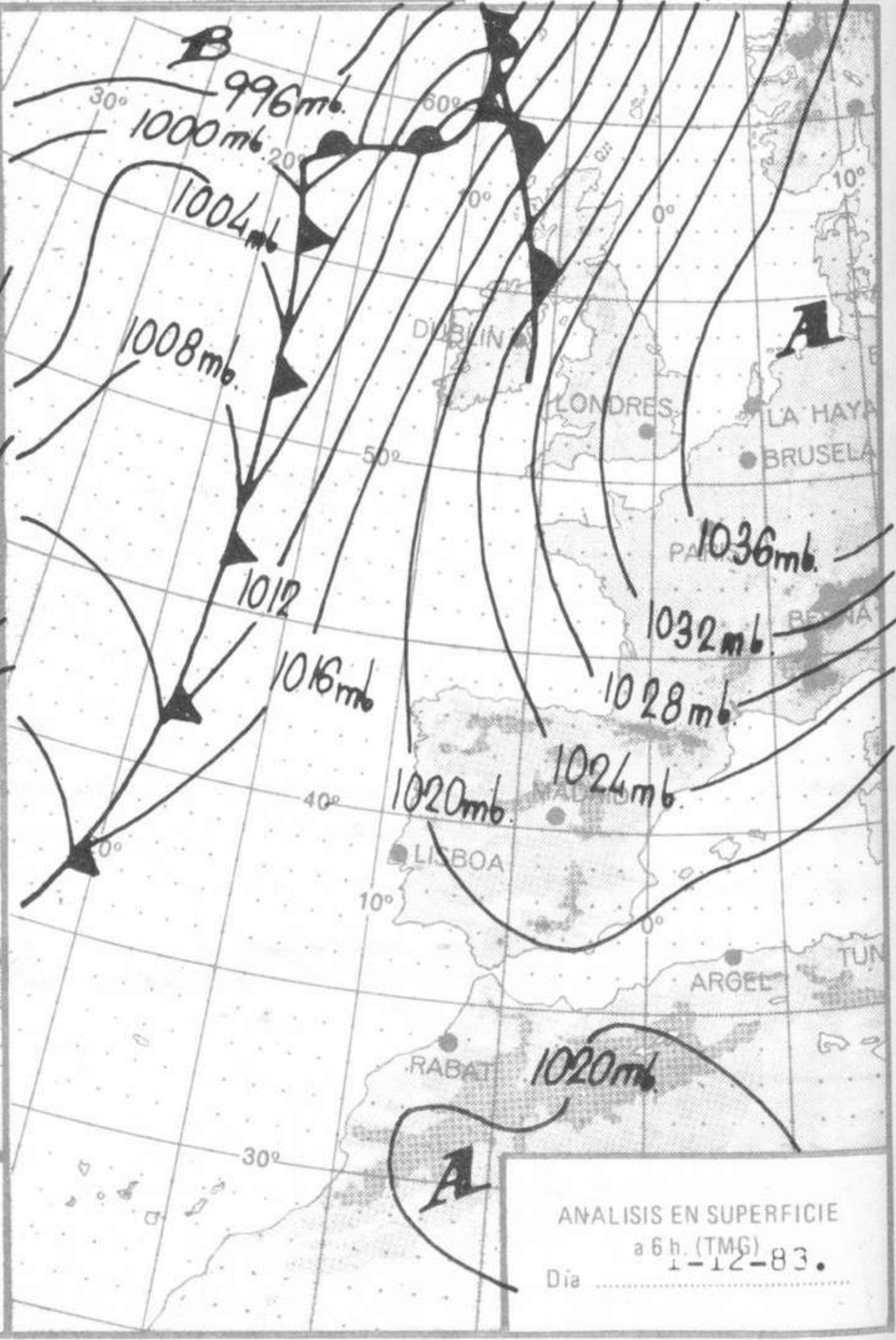
ANALISIS EN SUPERFICIE a 18 h. (TMG) Día 30-11-83
