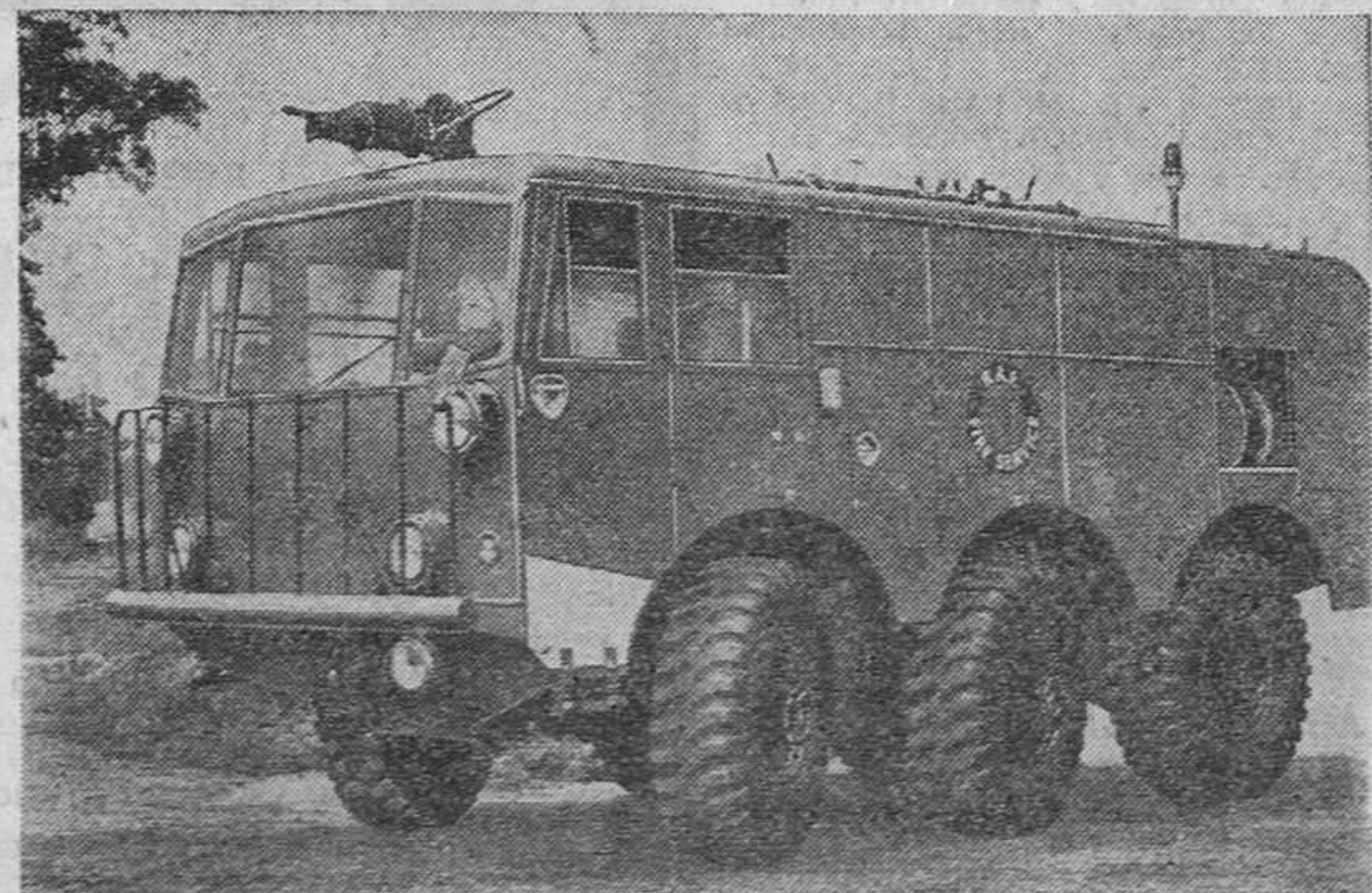
LONDRES.—Este tender contra incendios, que puede lanzar 22.729 litros de espuma por minuto, fué desarrollado para satisfacer las necesidades en los campos de aviación. Tiene dirección a cuatro ruedas y transmisión a seis, y ha sido diseñado para superar las dificultades que se encuentran en terrenos accidentados y pantanosos. El surtidor, montado sobre la cabina de conducción, lanza la espuma a más de 36 metros de distancia. — (Foto Capfe.)
