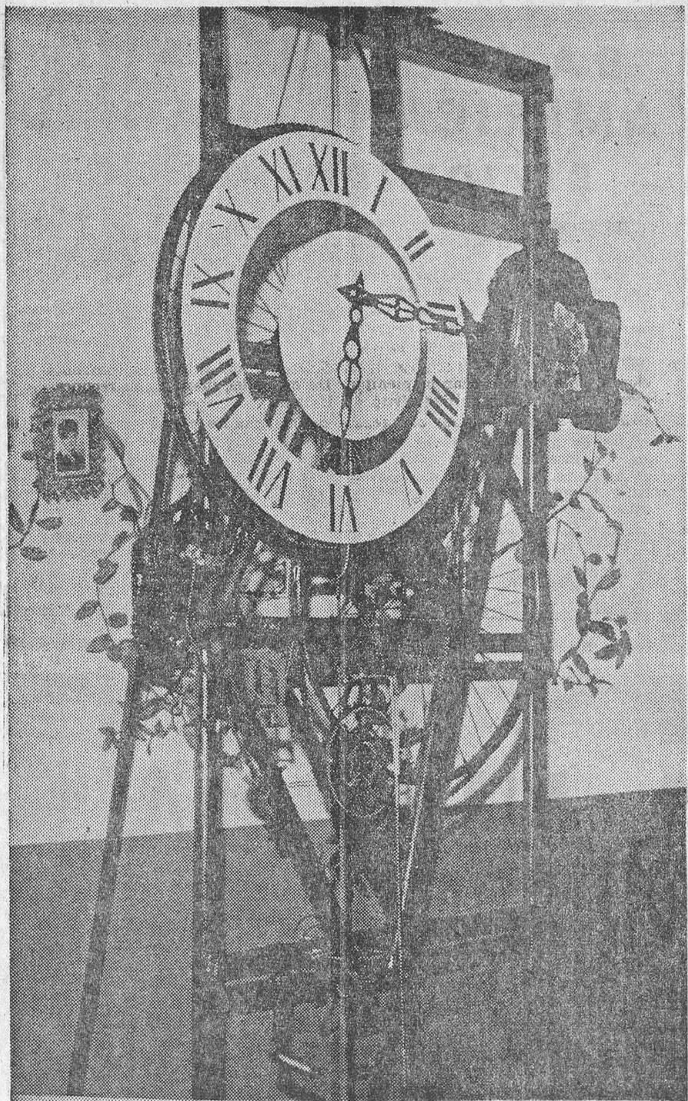
Don Francisco Escalont, carpintero de Arteijo (La Coruña), ha construido con piezas de una bicicleta que había comprado por doscientas pesetas, este gigantesco reloj, que funciona con elementales engranajes y un peso de veinticinco kilos
