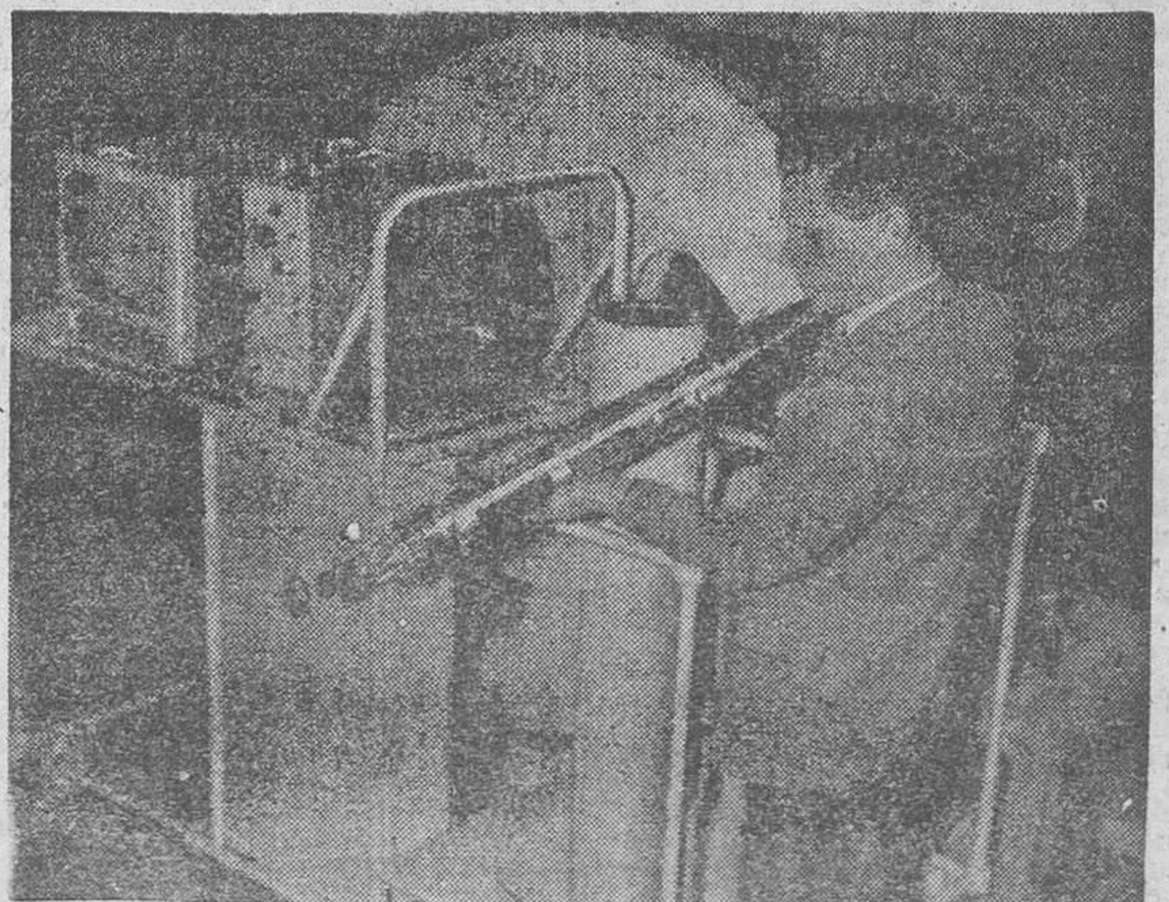
Una firma británica de ingenieros electricistas ha producido un nuevo tipo de cámara de televisión que, colocado dentro de un horno de reactor atómico, transmite su funcionamiento mientras el reactor se encuentra radioactivo. En esta fotografía, un ingeniero sostiene la cámara en la mano y al fondo se ven los controles y el aparato receptor montados en un trole. La cámara, que mide 76 cm. de largo, está protegida por una envoltura de acero inoxidable. (Foto Calpe)
