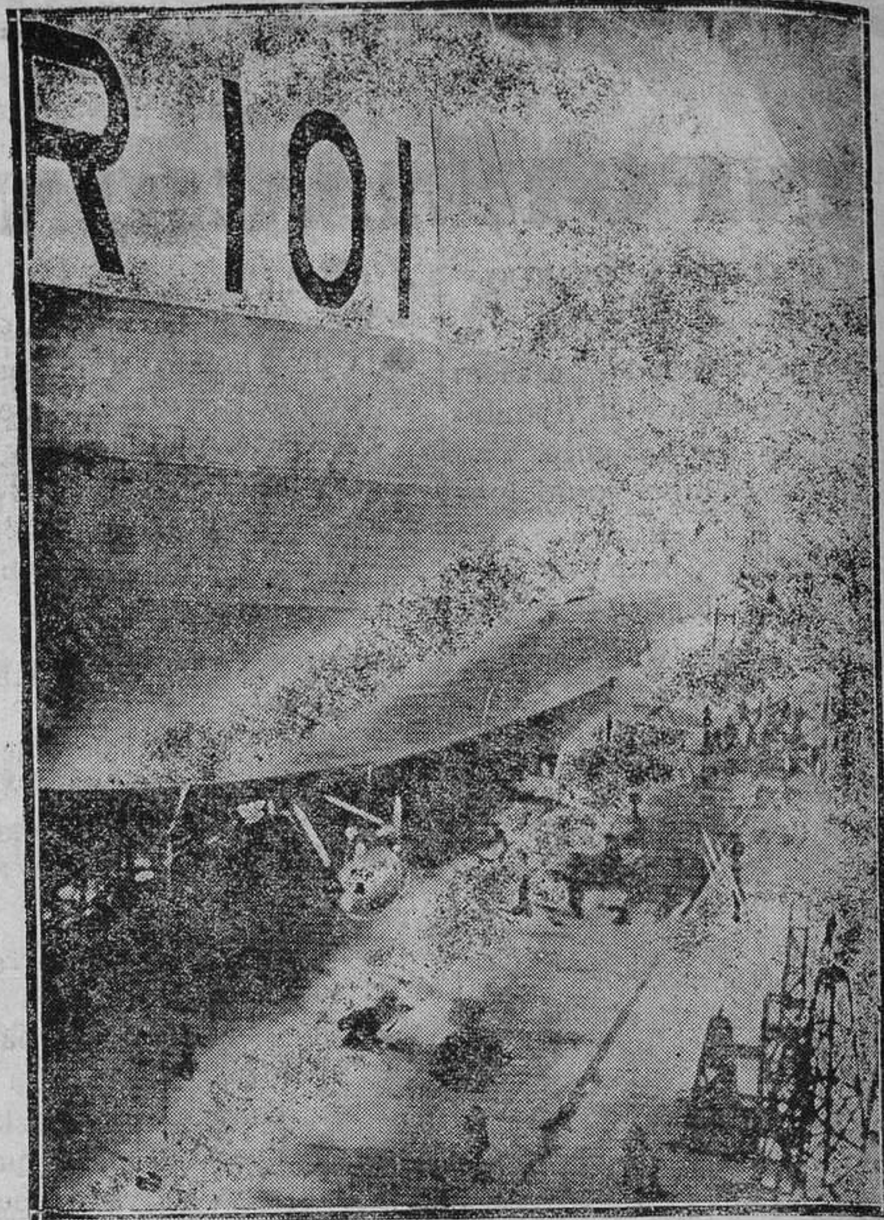
LONDRES.— El dirigible gigante "R. 101", en su "hangar" de Cardington. Este gran aparato, mucho mayor que el "Graf Zeppelin", mide 220 metros de largo, 49 de ancho, 40 de diámetro máximo, teniendo una capacidad total de 141.000 metros cúbicos. Puede transportar unos cien pasajeros.
