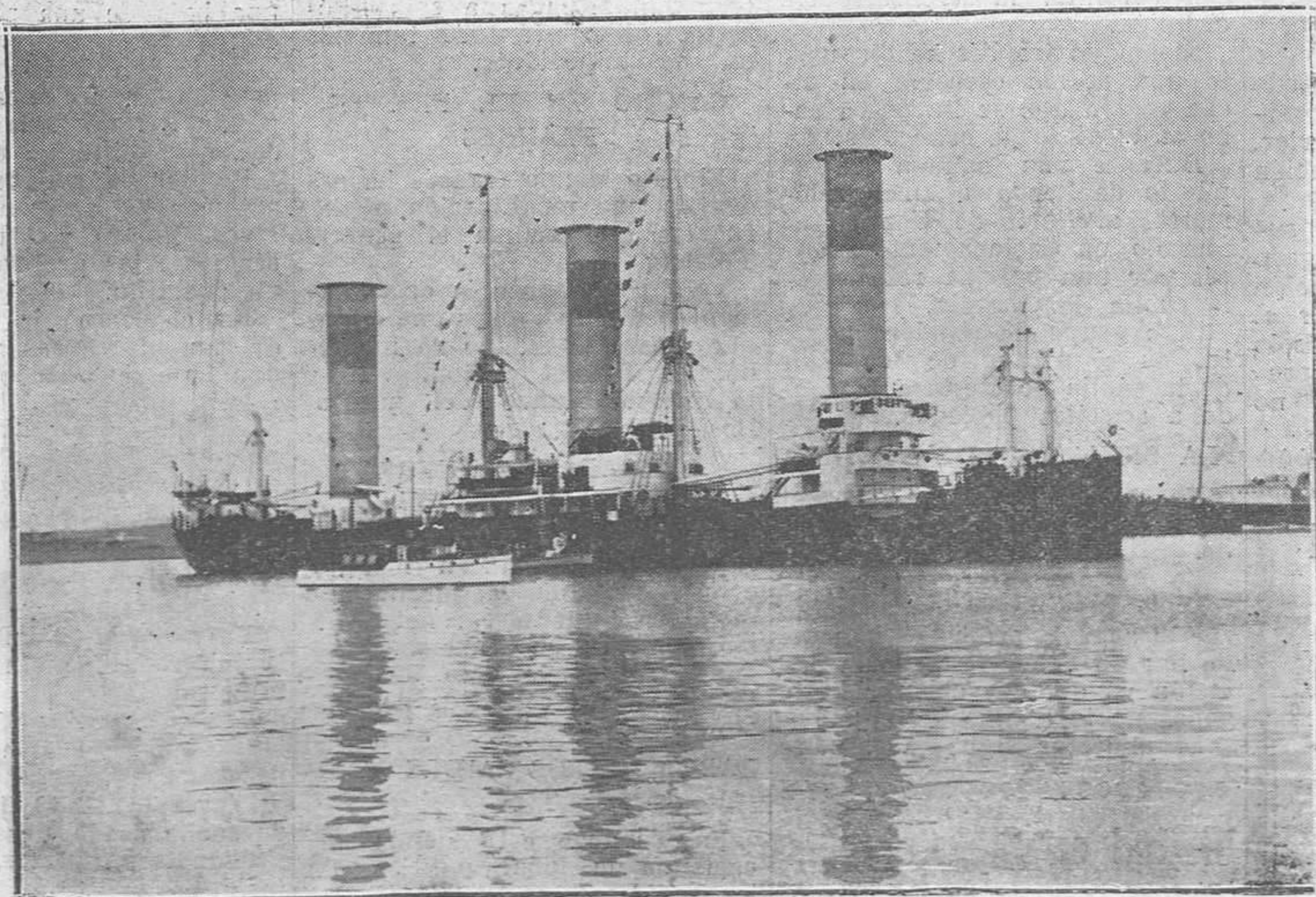
SANTANDER.-El buque rotor "Bárbara" alemán, que ha entrado en la bahía. La llegada de este buque ha despertado la curiosidad, pues los principios en que se funda el invento da lugar a apasionados comentarios. (Foto Samot)
