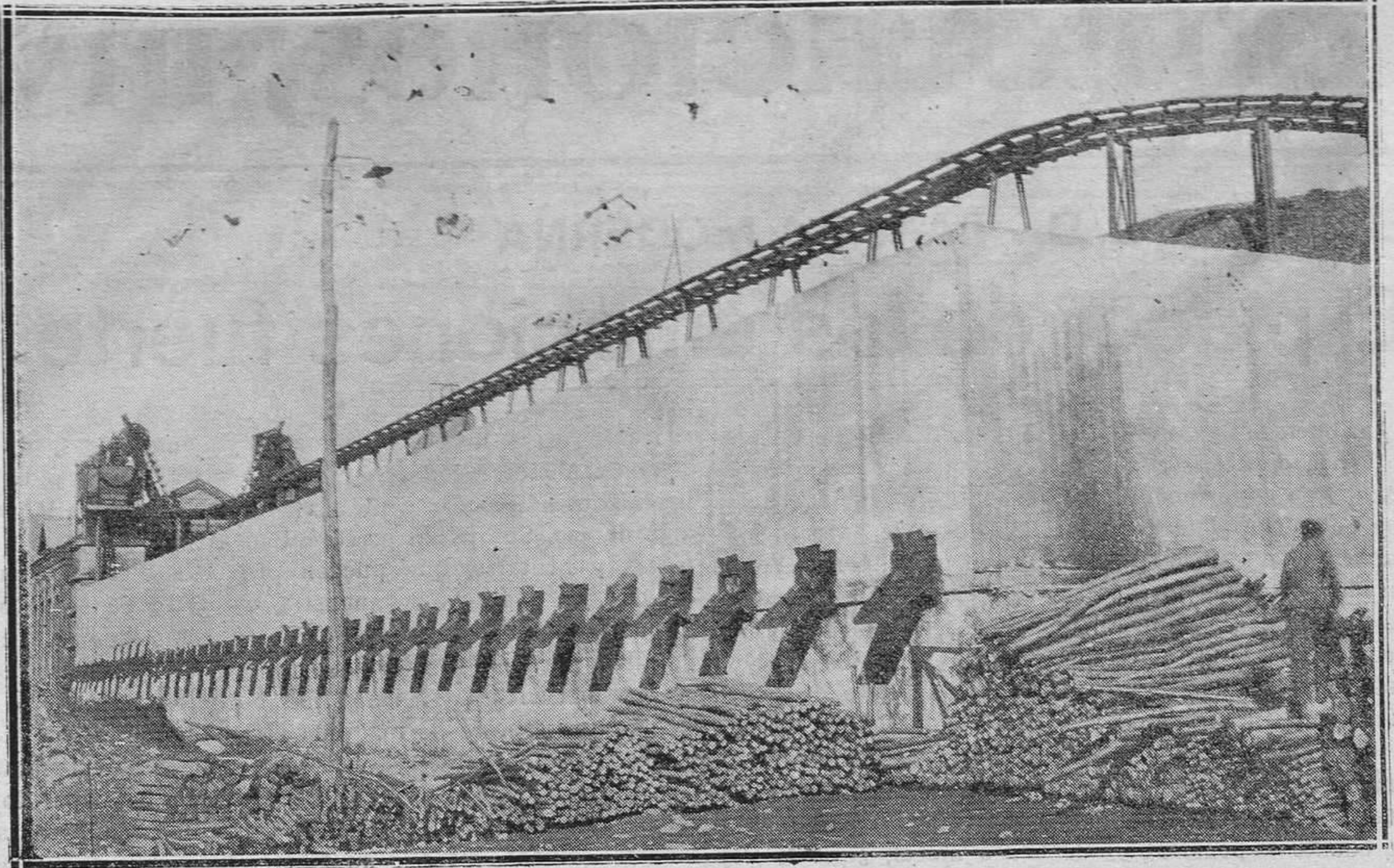
DE LA FABRICA DE MIERES.-Tipo de cargaderos de carbones, de los que hay ya construídos y en construcción.
