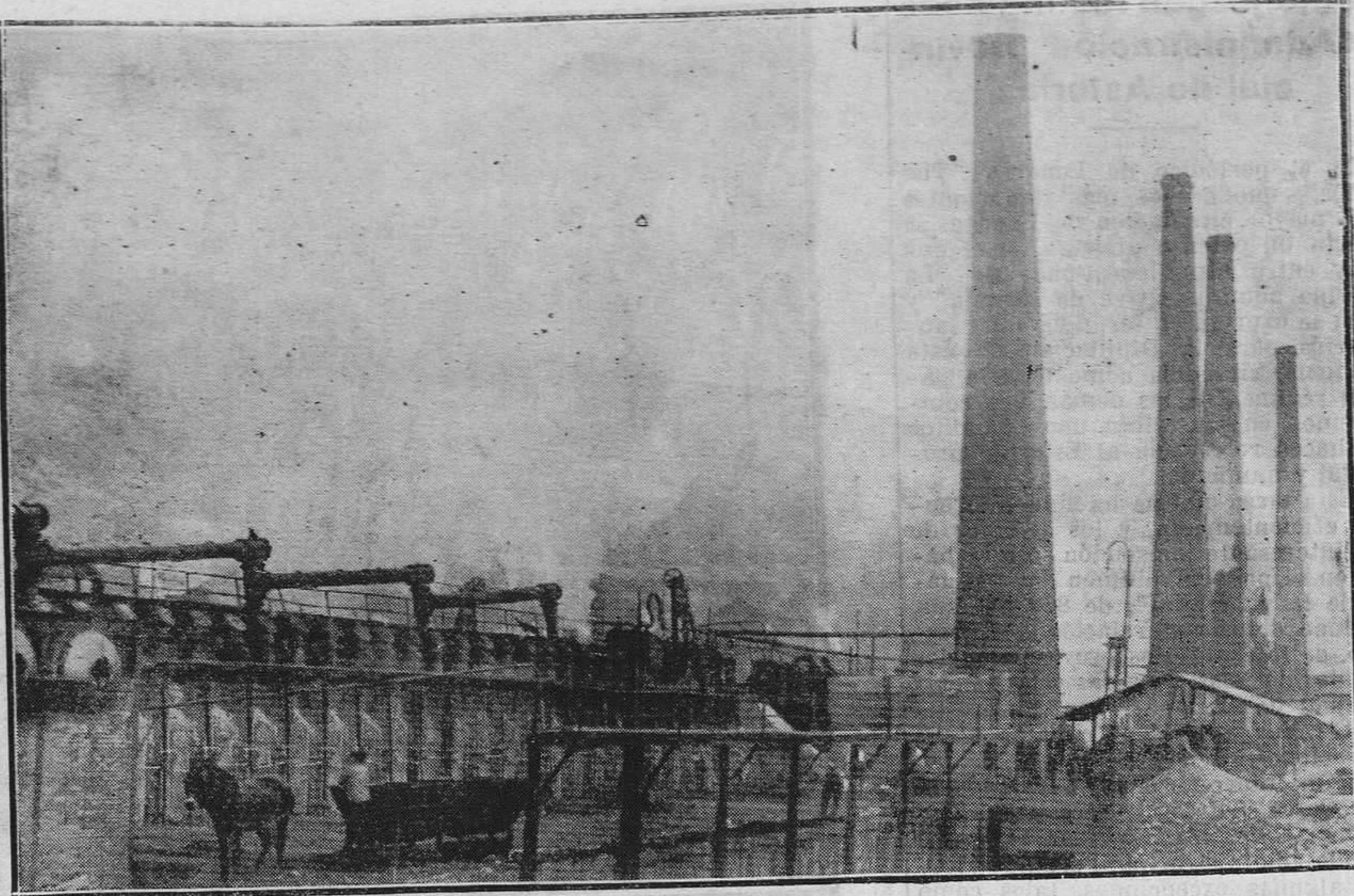
DE LA FABRICA DE MIERES.-Importante batería de doce hornos de cok, y a la vez generadora de importantes productos químicos.
