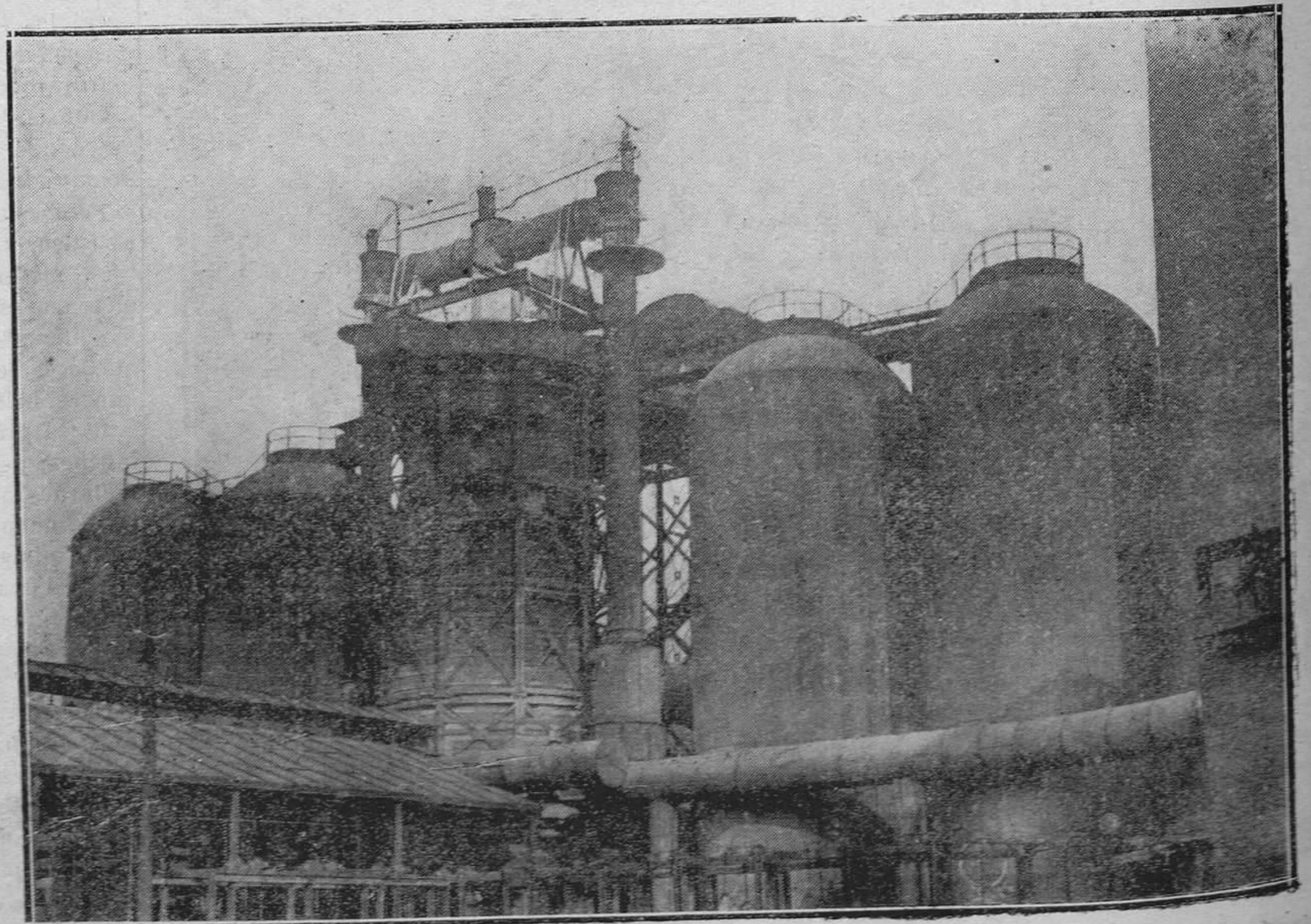
DE LA FABRICA DE MIERES.-Alto Horno. número 1, en el que se aprecian las estufas Cooder
