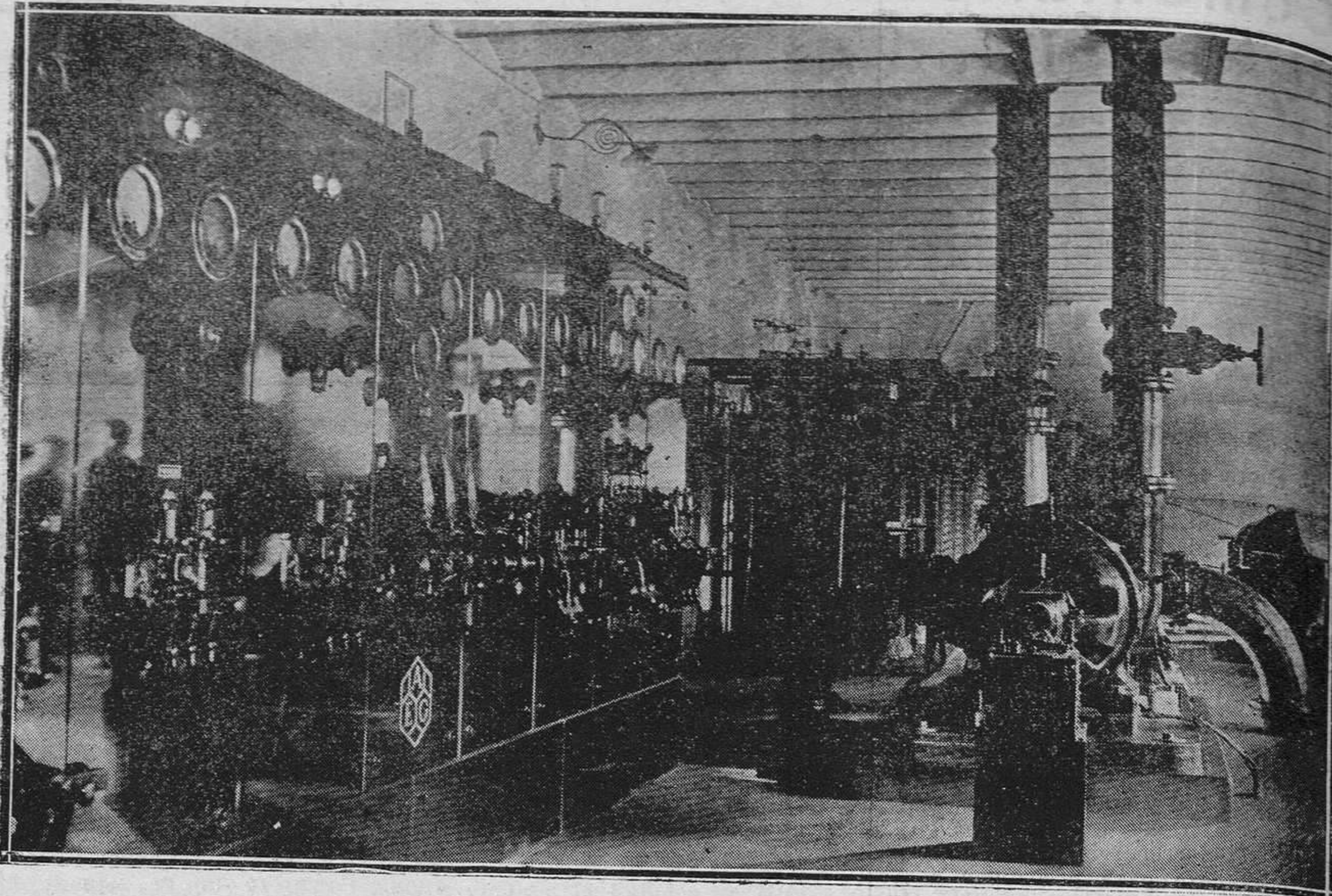
DE LA FABRICA DE MIERES.-Interior de la sala de bombas, en el Barredo, cerca del Grupo "Baltasara".
