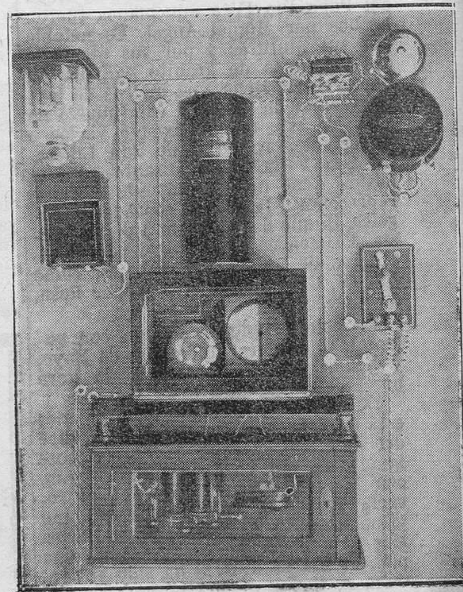
EL PRESISMOFONO UNCANIA. --Aparato inventado por el profesor de Química, de la Universidad de Bolonia, Dr. Emilio Uncania, y por medio del cual se perciben las perturbaciones sísmicas y se conoce la proximidad de un terremoto, con 24 horas de anticipación. El Presismofono, hace funcionar durante 30 segundos, una potente sirena.
