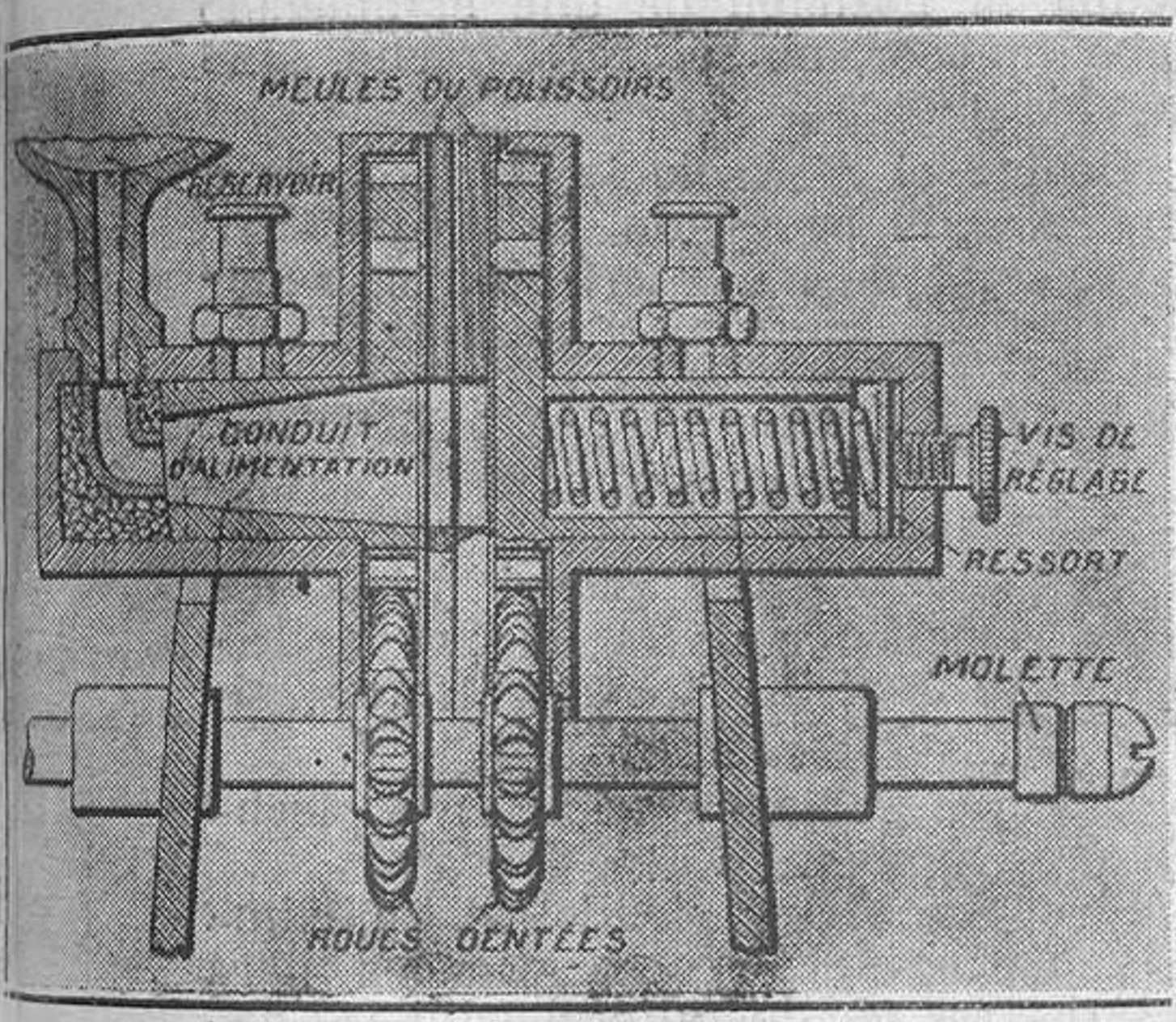
Máquina para pulir y afilar hojas de cuchillo.-Corte de la máquina
