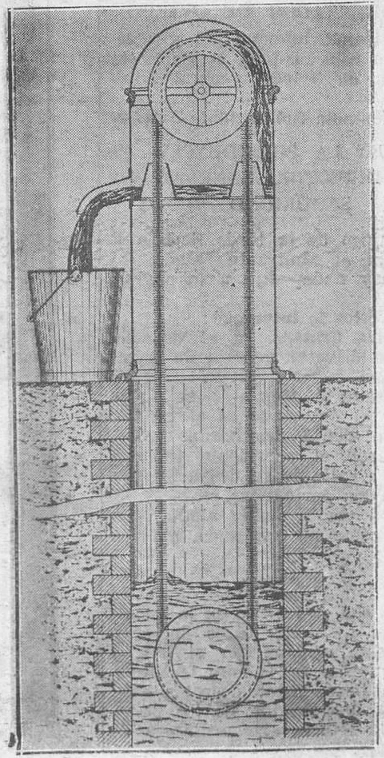
Instalación de una bomba en un pozo.
