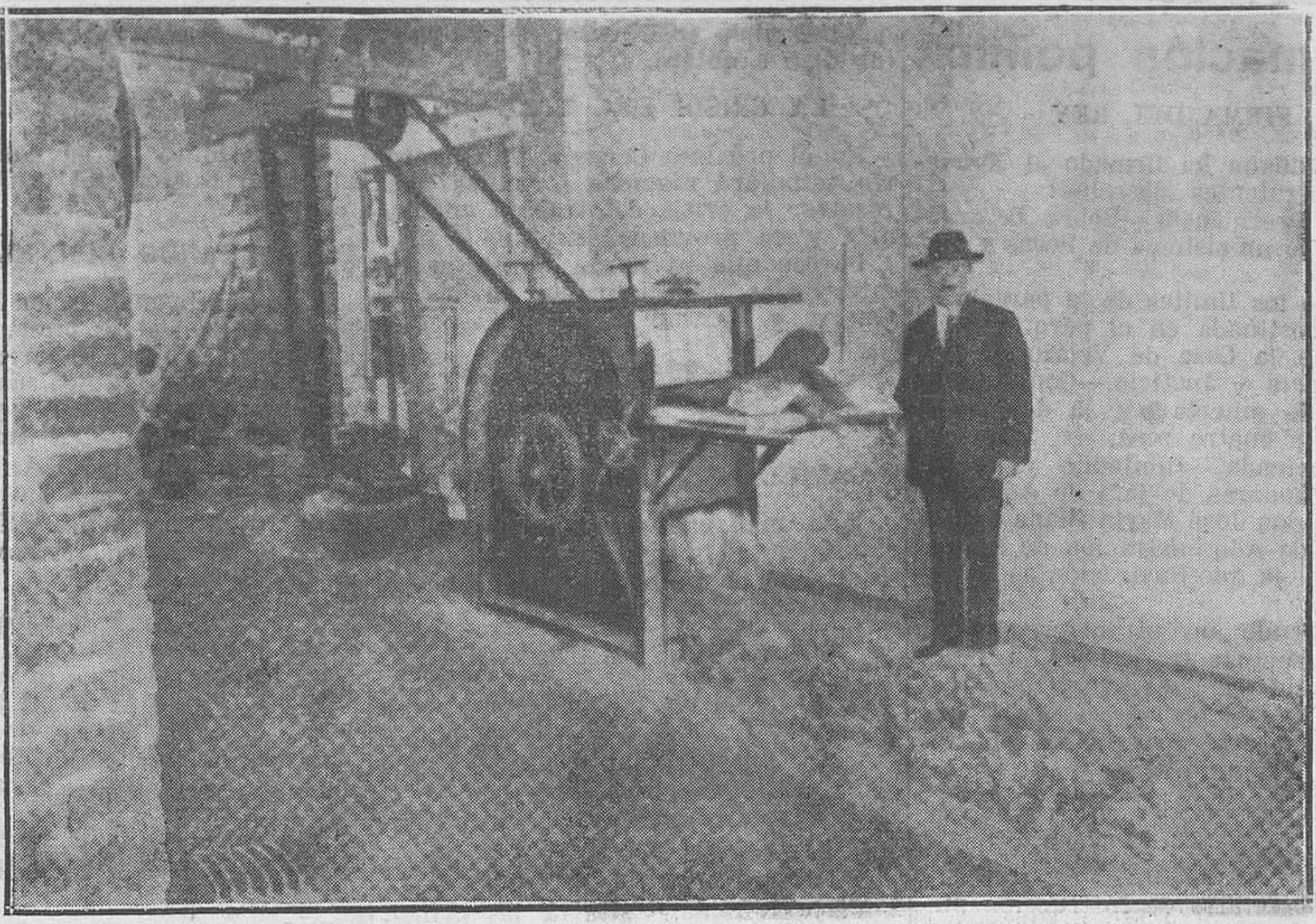
Vista de conjunto de una máquina nueva para extraer las fibras de las plantas textiles.
