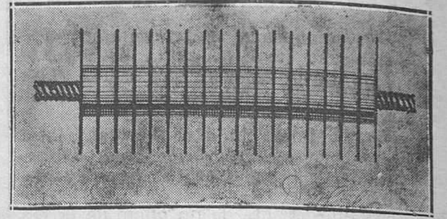
Detalle del cable de "cable-bomba", en el que se ve claramente la disposición de las rodajas metálicas y las rodajas de caucho.
