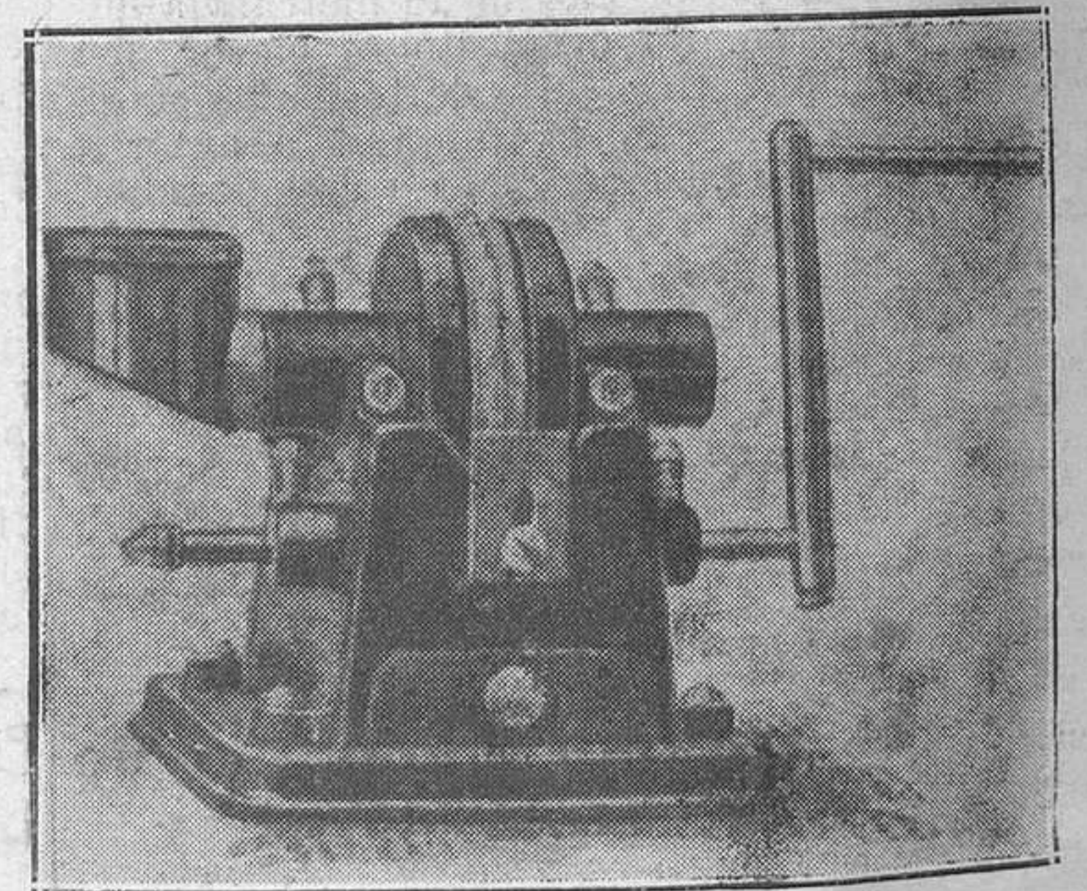
Máquina para pulir y afilar hojas de cuchillos y herramientas planas. Aspecto exterior.
