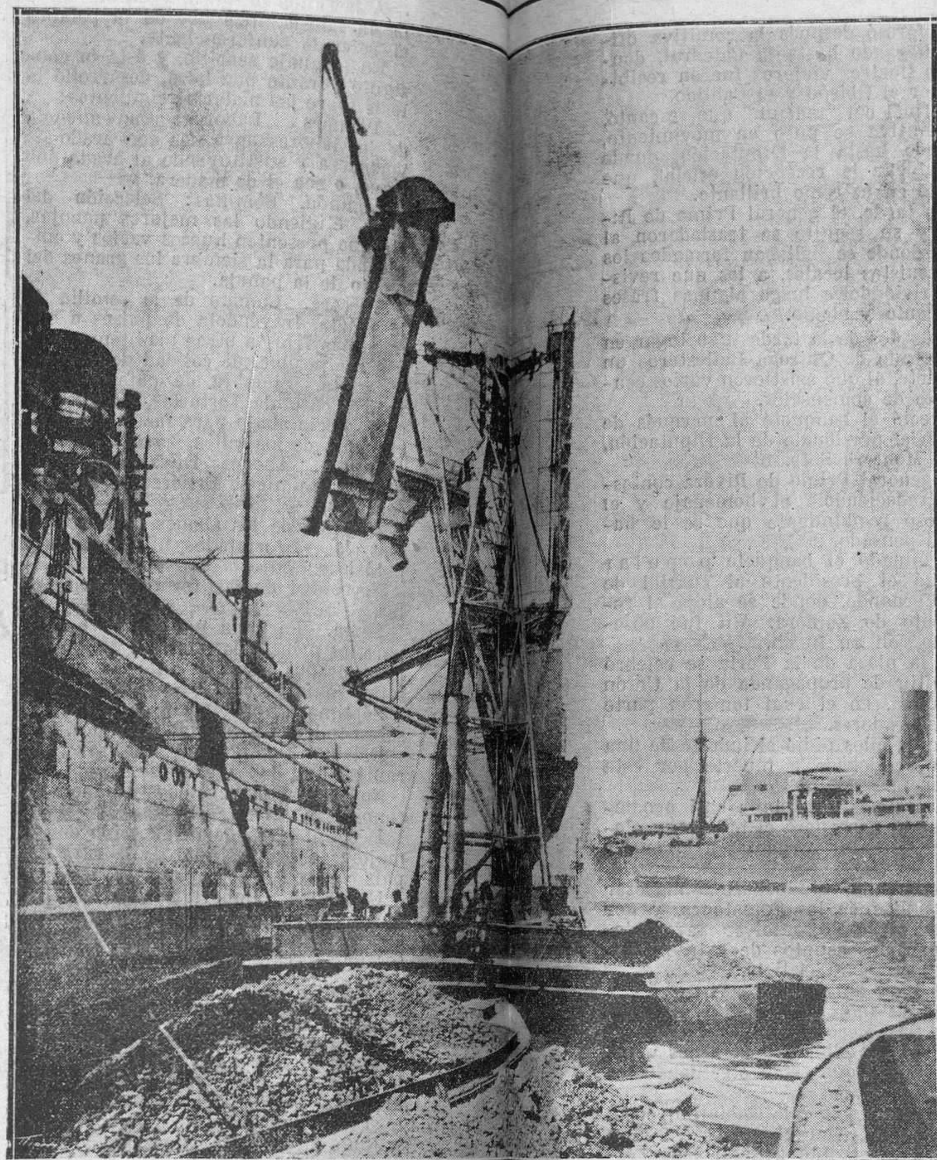
Instalación flotante que en el puerto de Hamburgo abastece de carbón a los buques por ambos costados a la vez.
