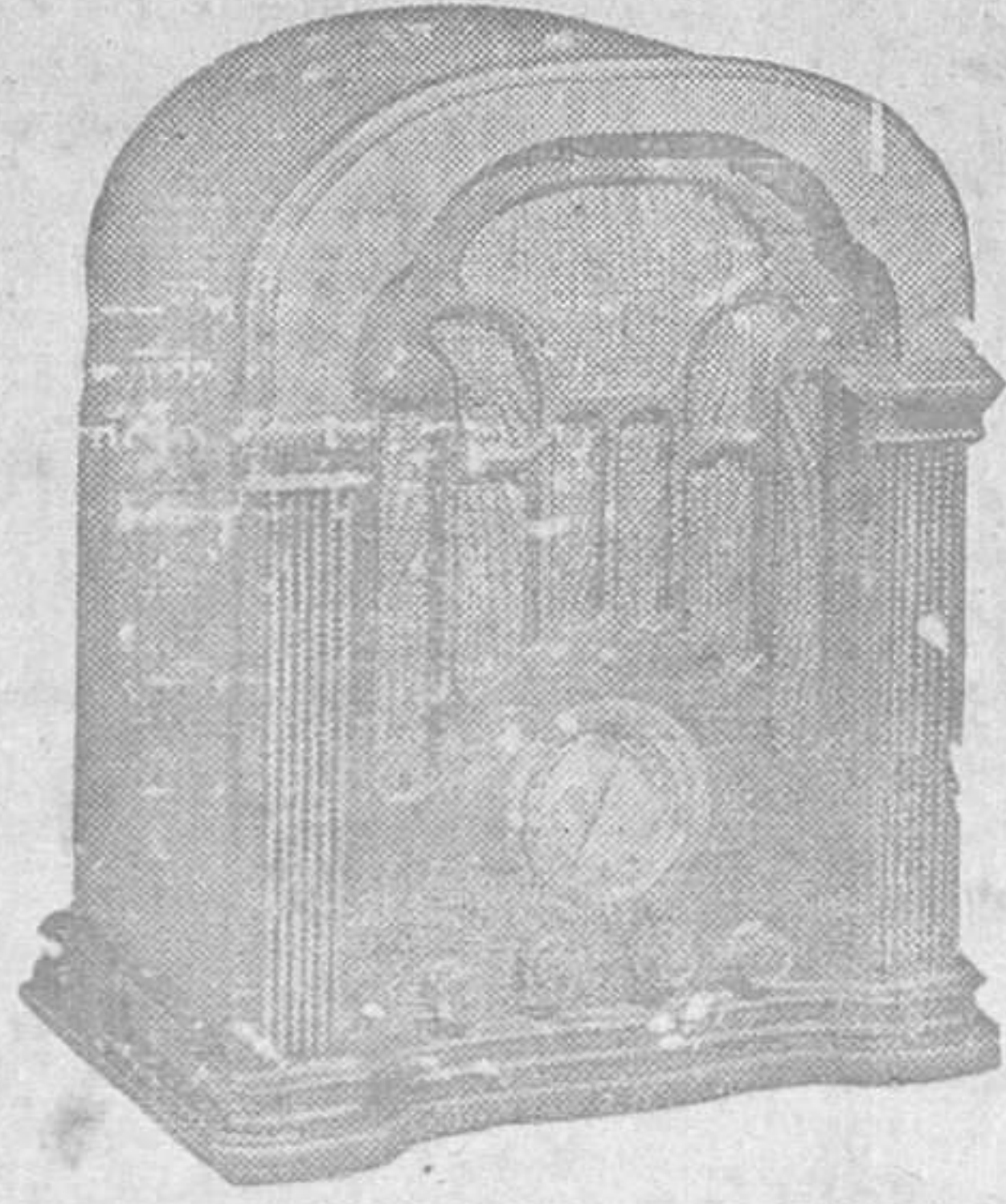
Superheterodino 6 válvulas, todas las ondas, seis circuitos sintonizados
