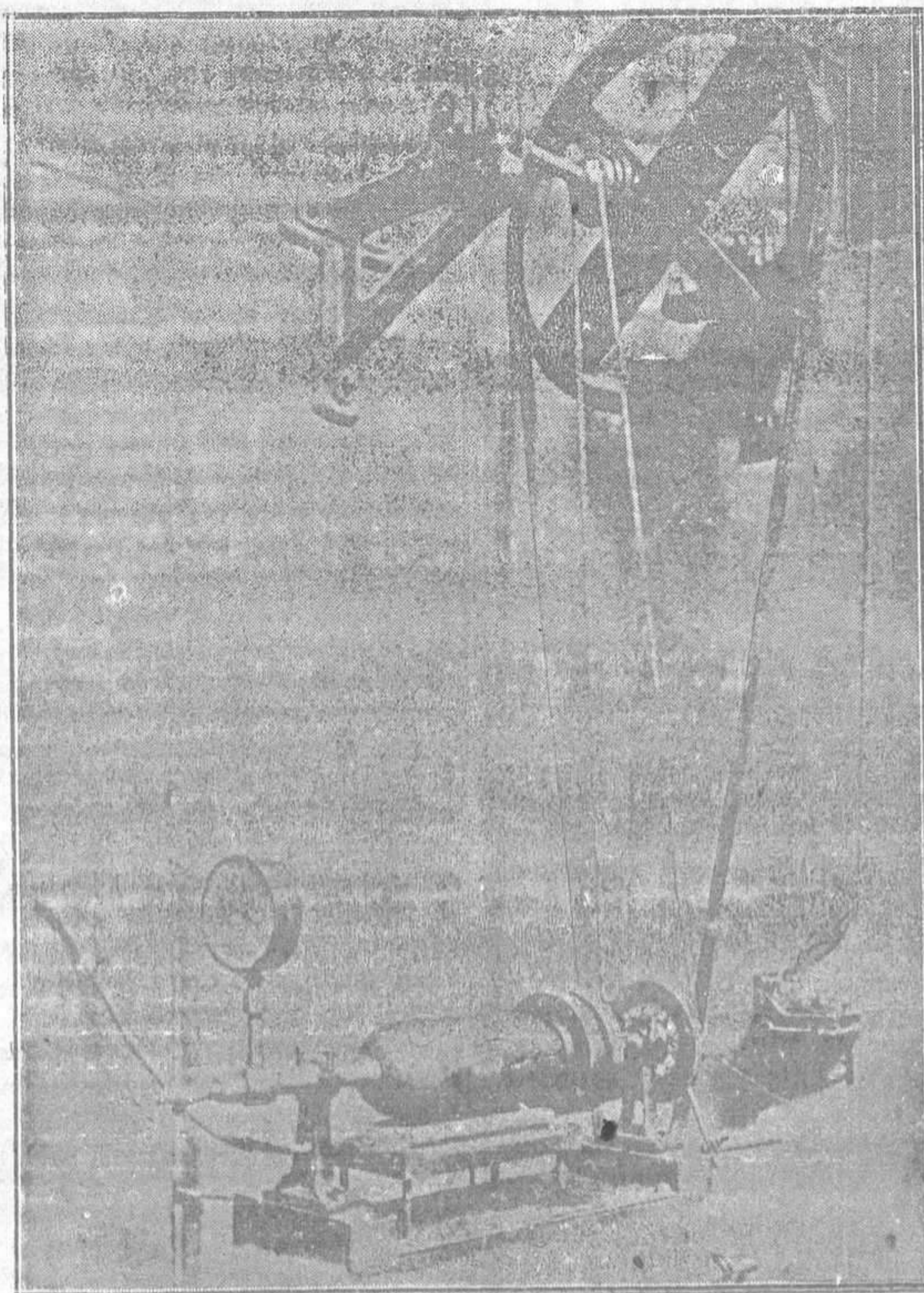
Bomba «Bergius», para la obtención de petróleo sintético
