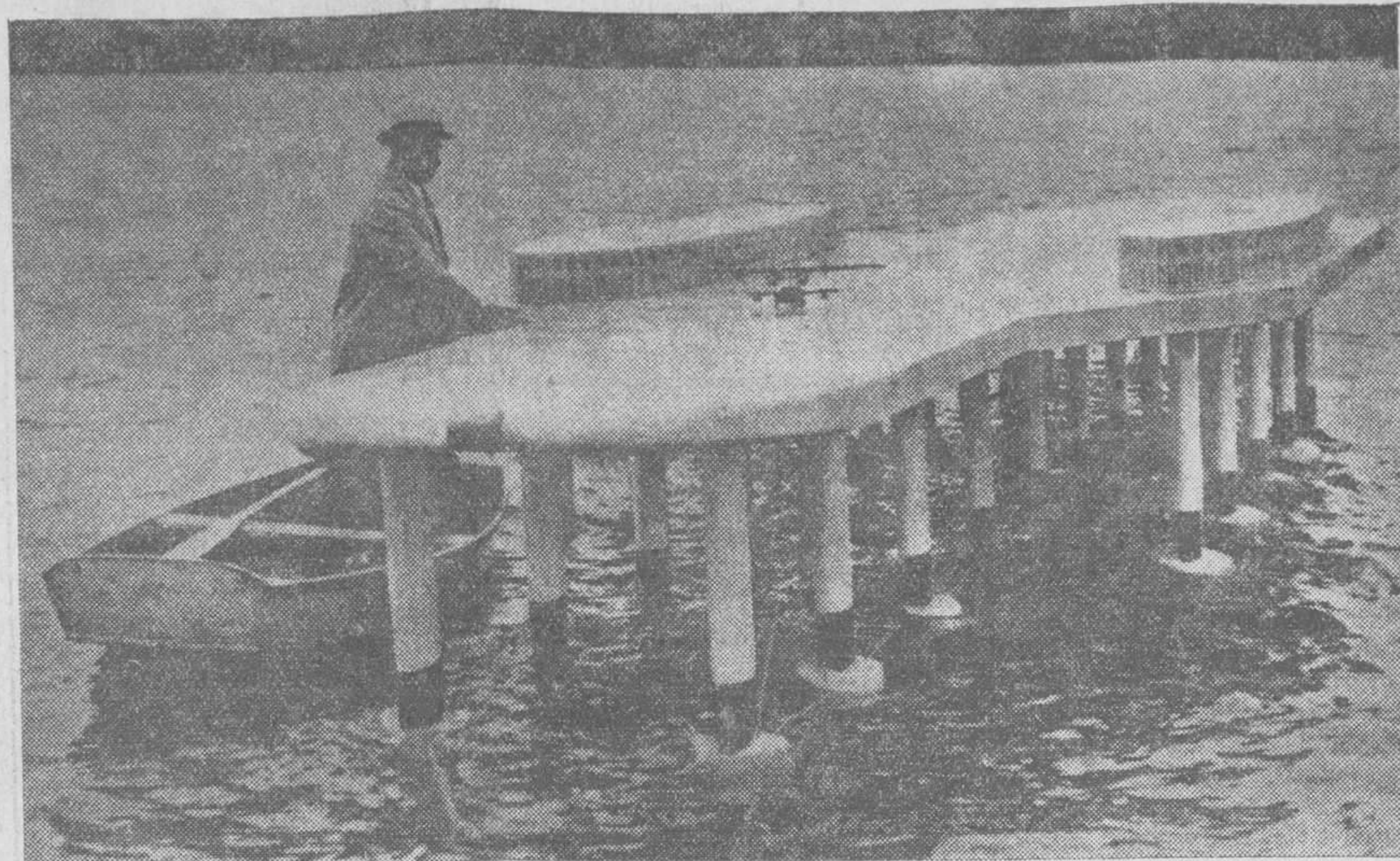
Modelo reducido del aeropuerto flotante ideado por el ingeniero norteamericano E. R. Armstrong, que se proyecta construir entre Nueva York y la isla Bermuda
