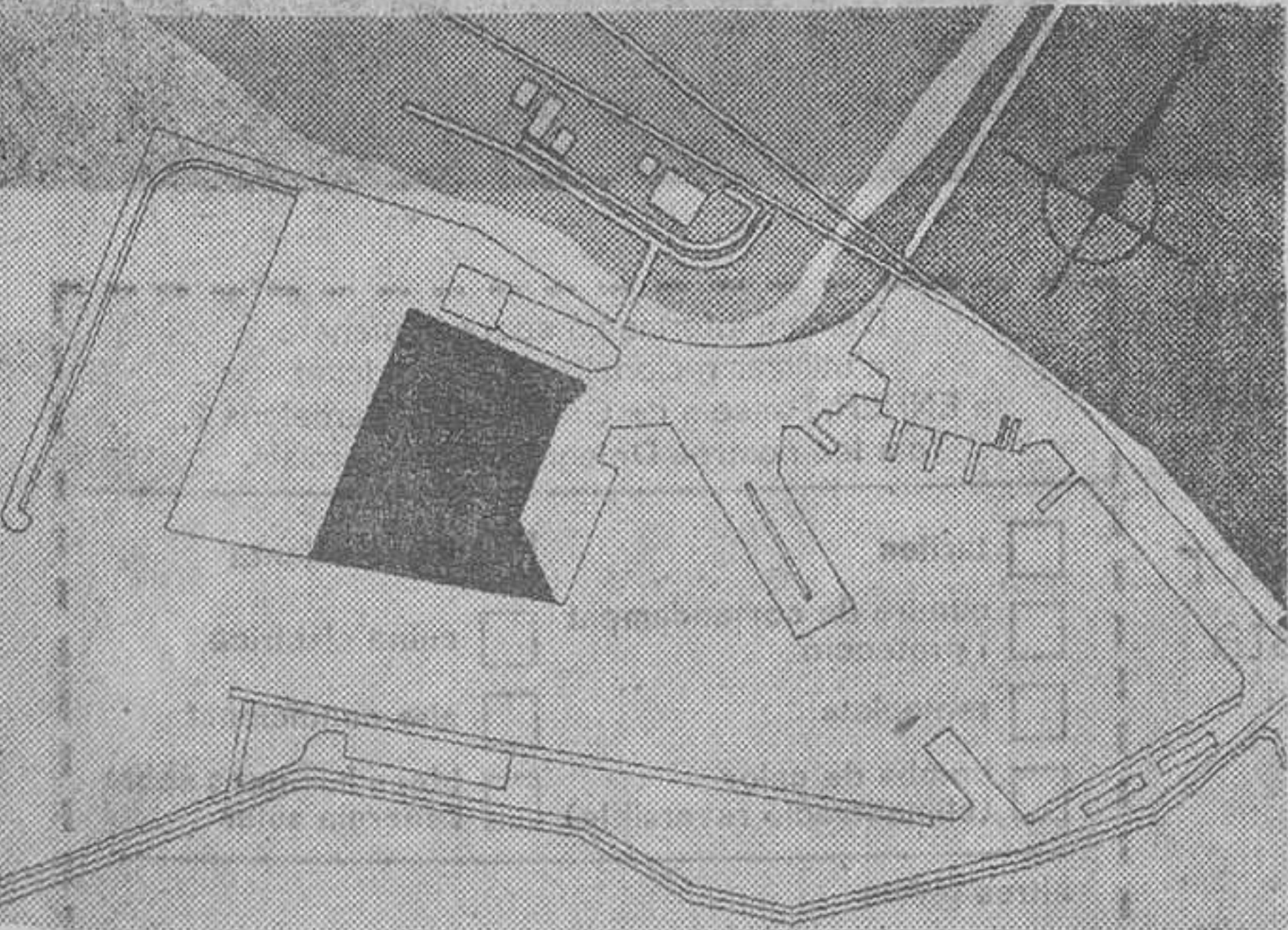
Plano general del Puerto de Tarragona. La zona oscura marca la superficie de las instalaciones de EXPOSA
