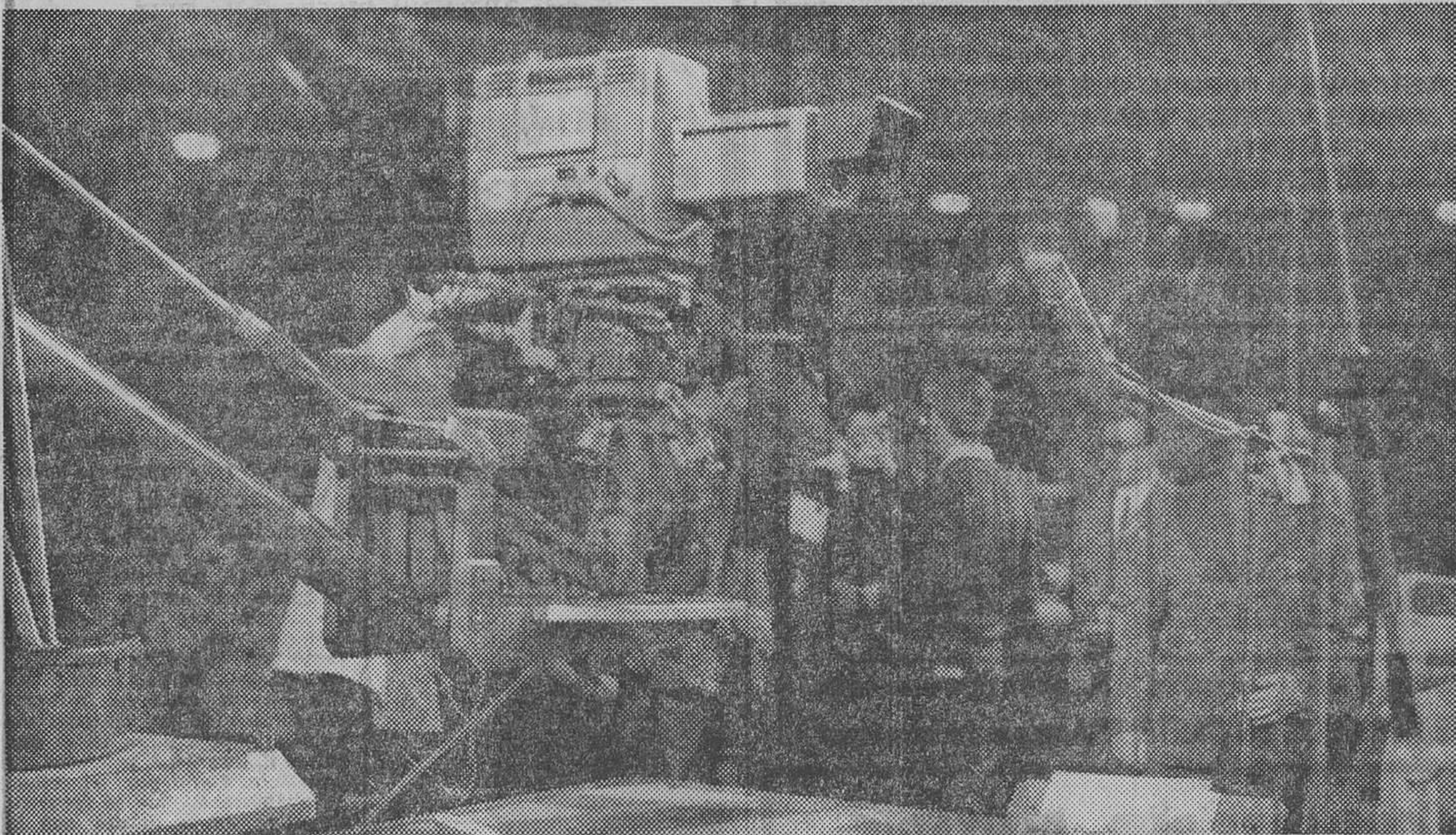
Una de las cinco cámaras «Philips-Plumbicón» para televisión en color, totalmente automáticas y transistorizadas, empleadas por T.V.E. en la transmisión internacional del Festival de Eurovisión.
