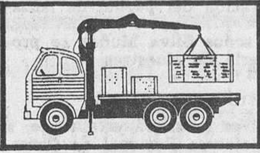
GRUAS SOBRE VEHICULO
