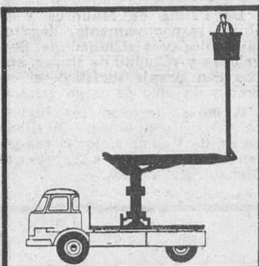
PLATAFORMAS SOBRE VEHICULO
