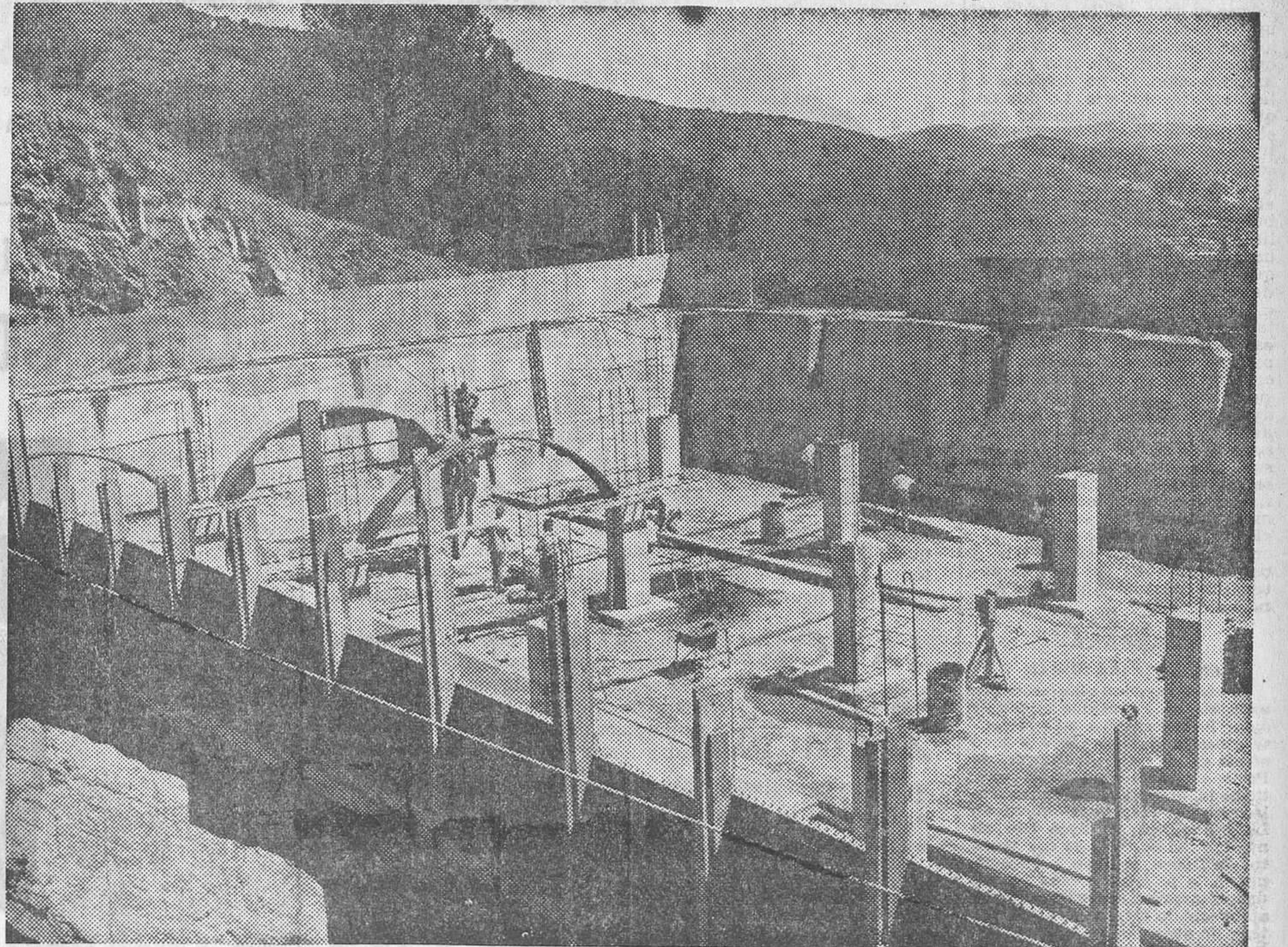
Una vista, captada a principios de mayo último, del hormigonado interior de muros y pilares del nuevo depósito regulador del servicio de abastecimiento de agua a Barcelona y que se está construyendo en la falda del Tibidabo, a la altura de la cota 260. Su capacidad es de dos millones de litros y está destinado al suministro de agua al barrio de San Ginés, en la zona NE de la ciudad. El depósito forma parte del plan de urgencia que está ultimando la SOCIEDAD DE AGUAS DE BARCELONA con vistas a la ampliación de sus instalaciones de distribución de agua potable
