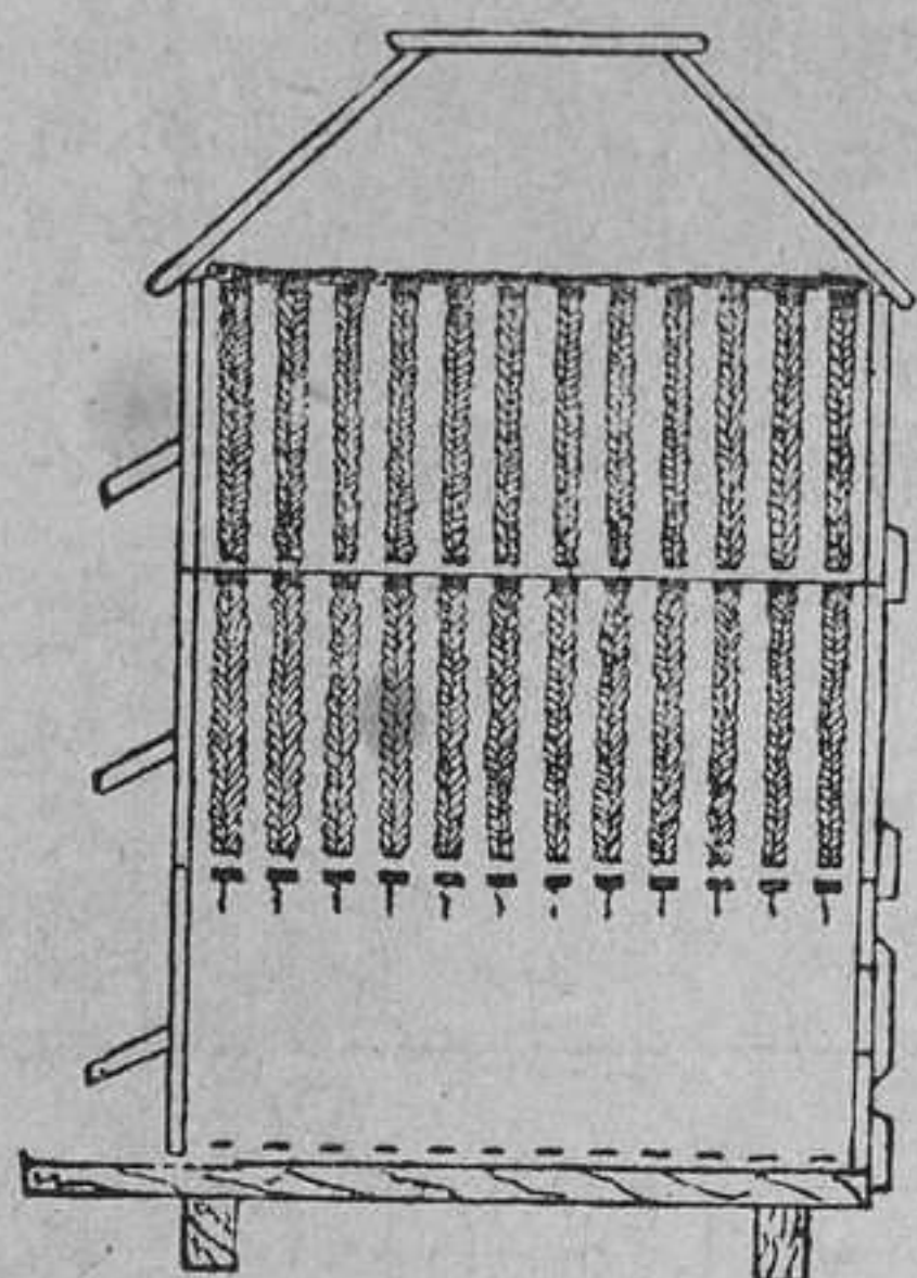
CORTE LONGITUDINAL DE UNA COLMENA "ECONÓMICA"
