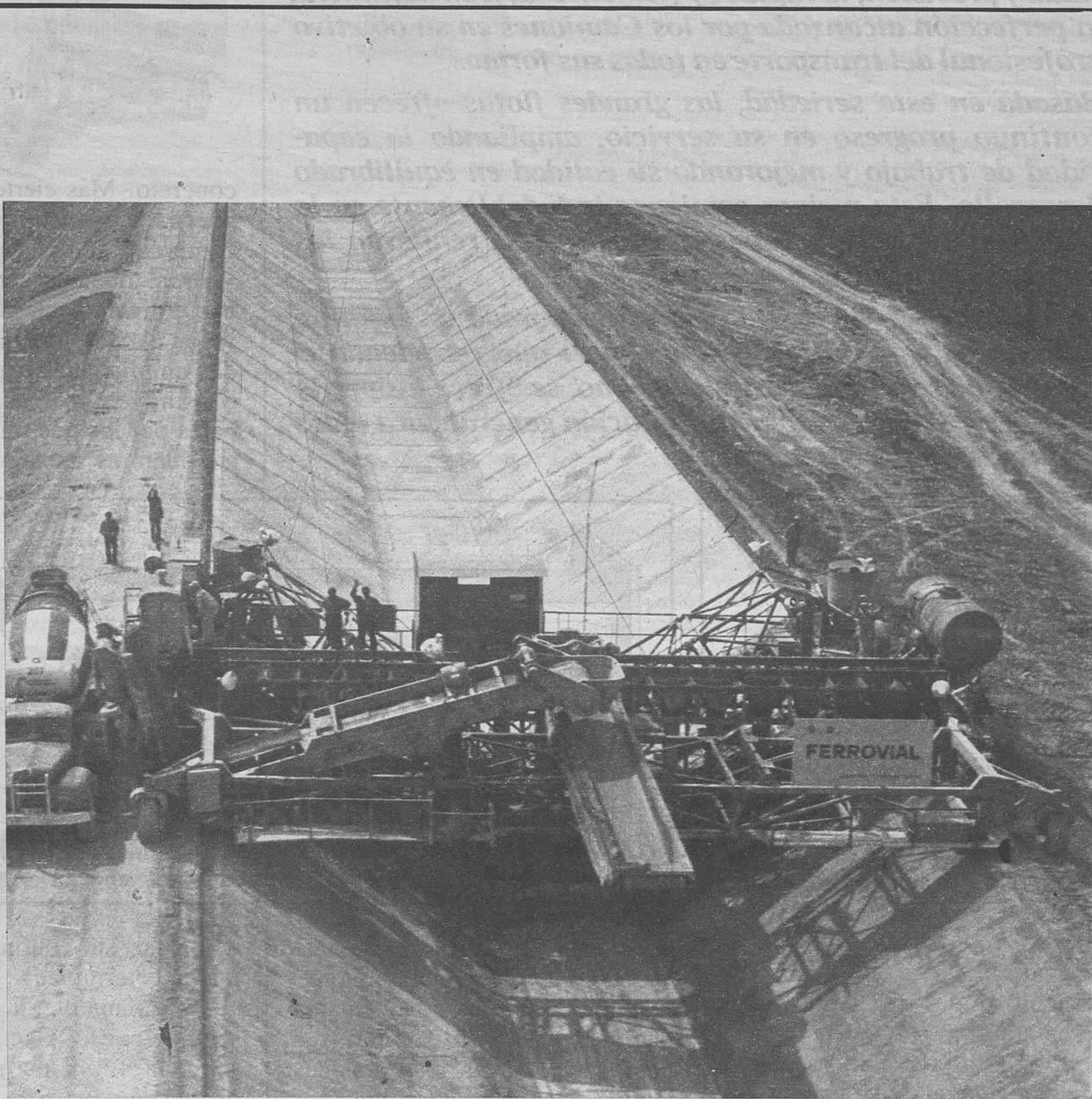
Canal de Fuensanta. Traslase Tajo-Segura
