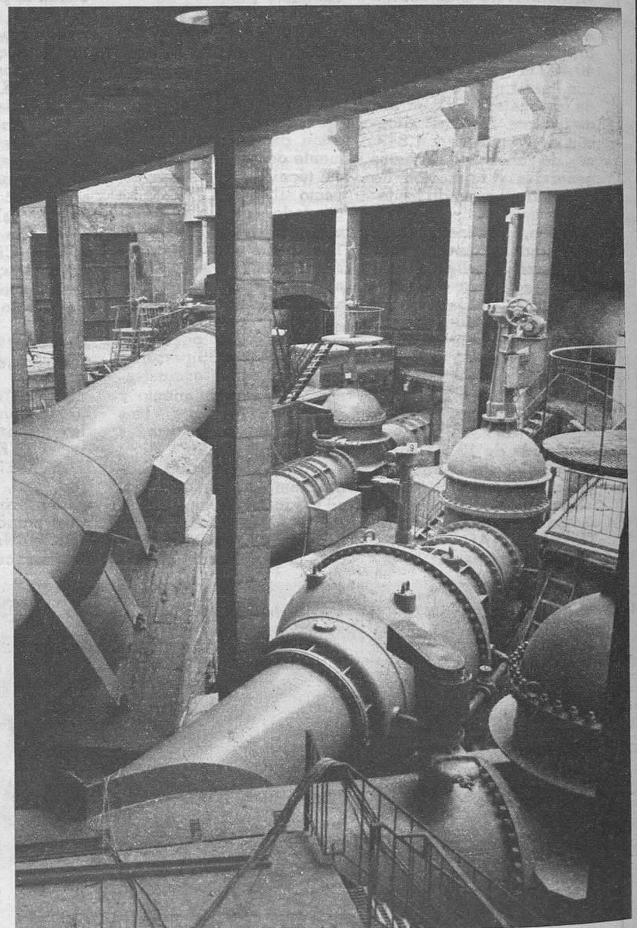
NUDO DE «EL GOLOSO»
