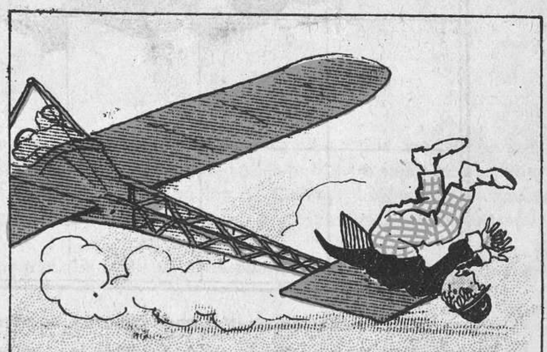
Como a quien nada le aterra y dijo saltando a tierra:
