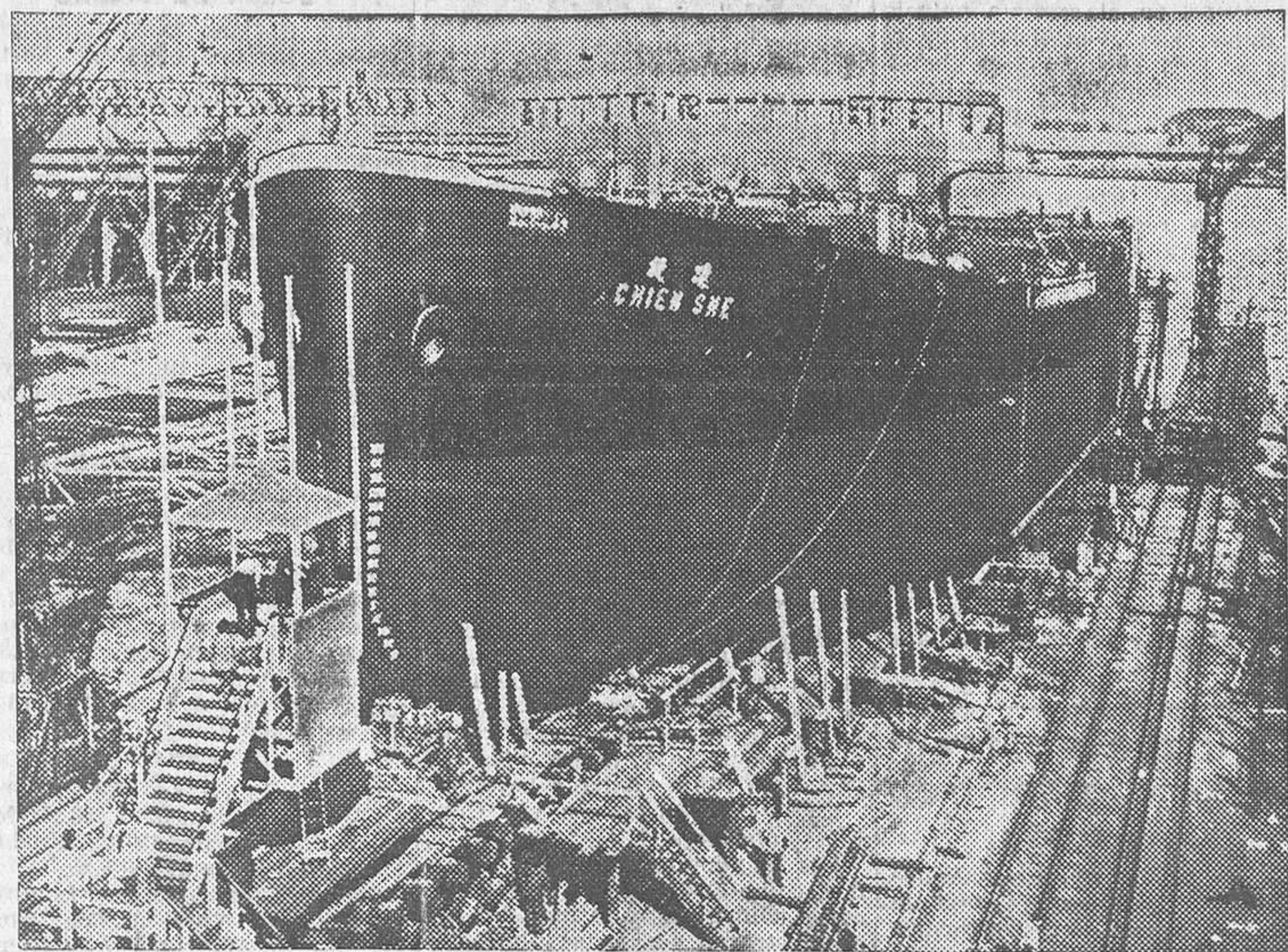
El mayor barco pesquero del Mundo, construido para el Gobierno de China y bautizado en Dantsig con el nombre de «Chien She»
