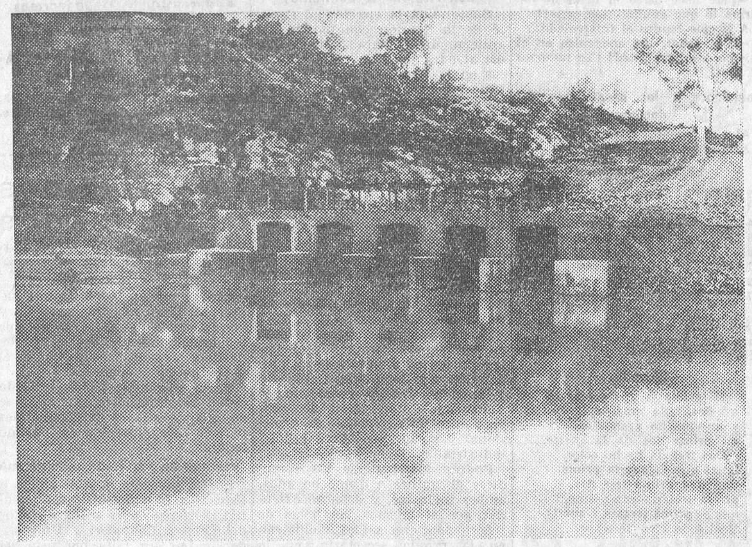
TOMA DE AGUA Y COMPUERTAS DEL SALTO DE CANAVEROSA. —Por esta toma atraviesa el río Segura la sierra llamada Serretilla, con una longitud de 1.900 metros
