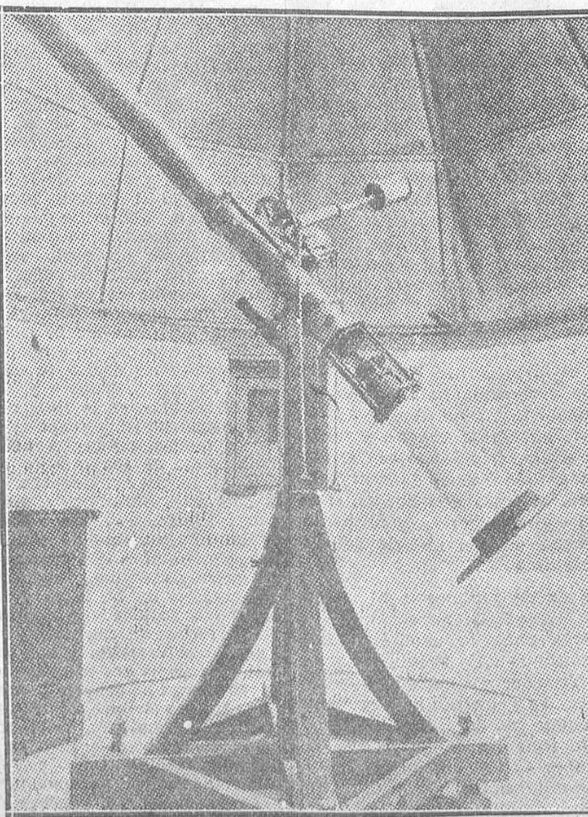
Heliógrafo de Zeiss, con el que se fotografian las manchas solares en el Observatorio de Madrid
